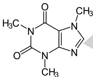
Struktur kimia kafein
