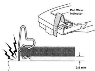
Gambar 50. Indikator keausan pad.
