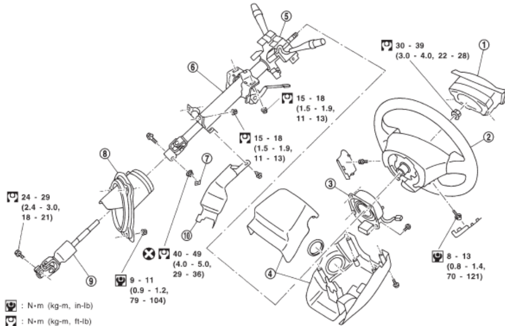
Gambar 200. Steering column.
