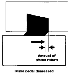
Gambar 52. Elastisitas seal.
