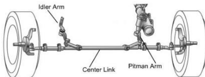
Gambar 133. Sistem kemudi tipe gear box suspense indipenden.
