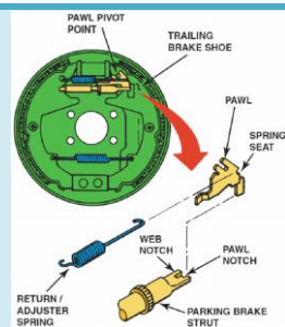
Gambar 28. Komponen penyetel roda bintang.
