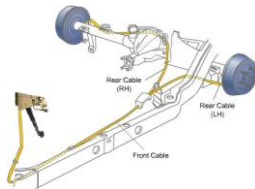
Gambar 38. Mekanisme rem parkir.
