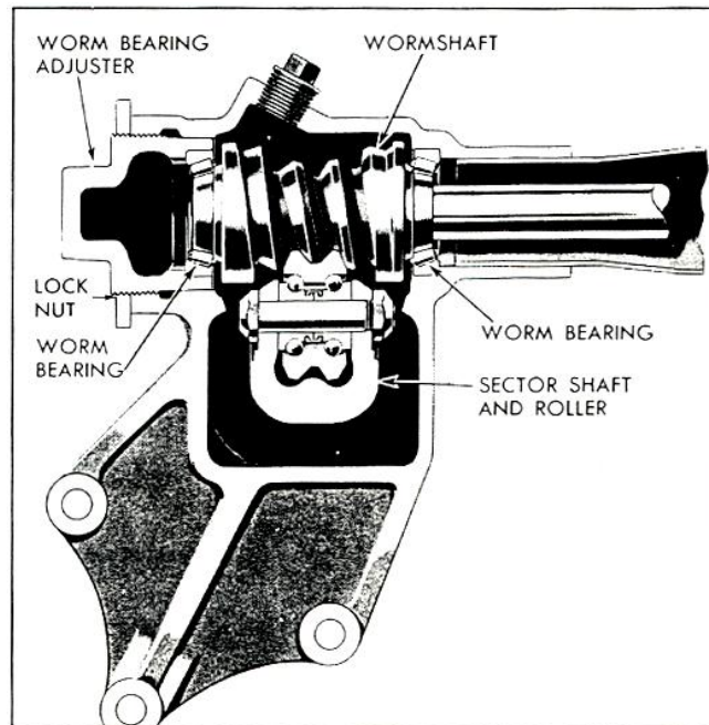
Bambar 189. Konstruksi roll and worm.
