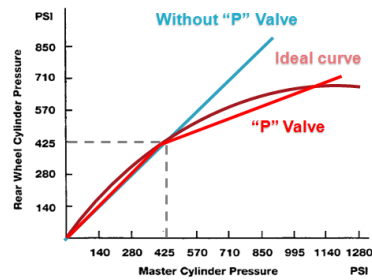
Gamabar 68. Grafik katup proporsional.
