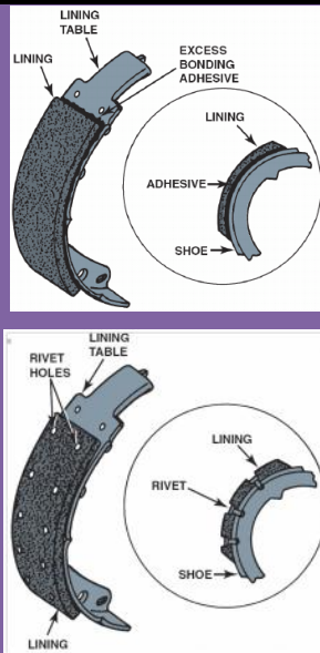
Gambar 9. Sepatu rem.
