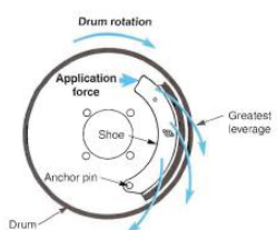
Gambar 31. Self-energizing effect pada sepatu rem primer .
