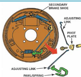
Gambar 26. Komponen penyetel roda bintang.
