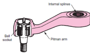
Gambar 141. Lengan pitman.
