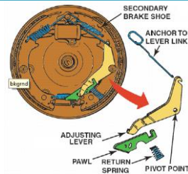
Gambar 27. Komponen penyetel roda bintang.
