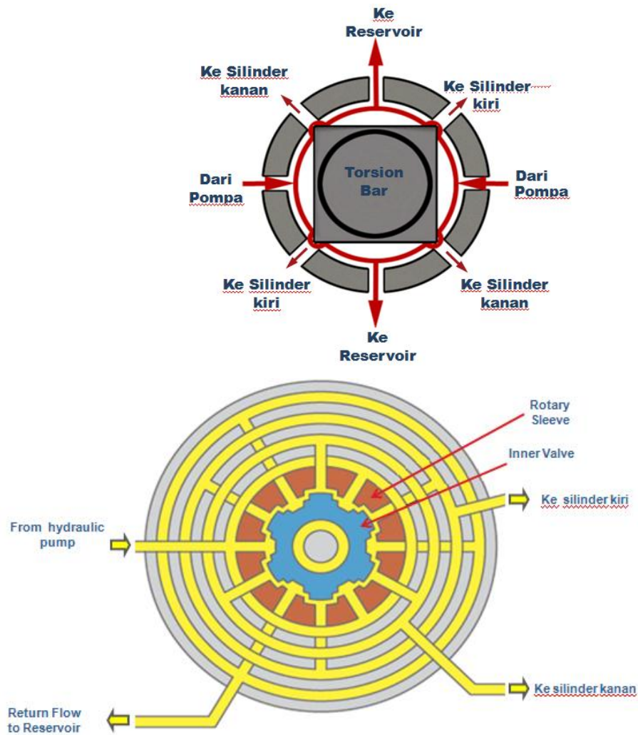
Gambar 166. Cara kerja control valve pada posisi lurus.
