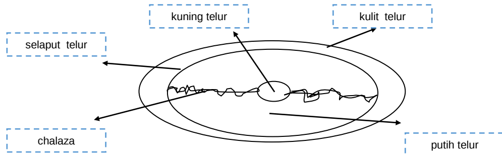
Gambar 9. Struktur Telur.
