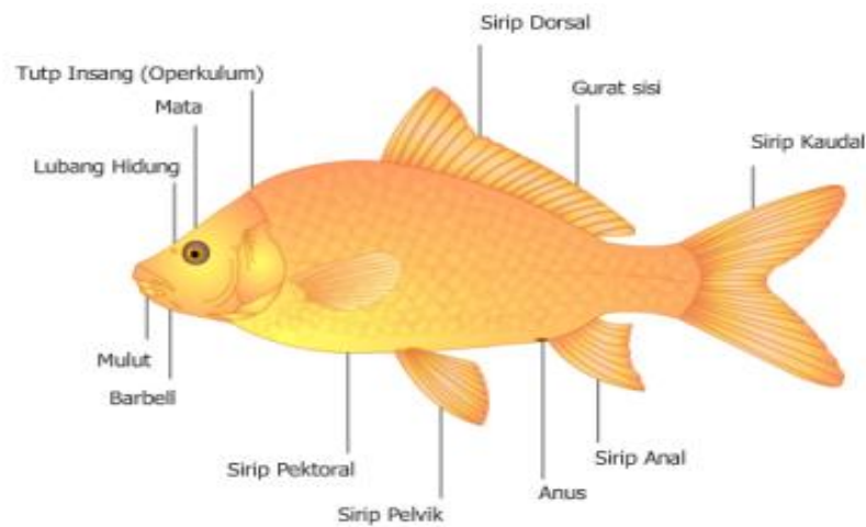
Gambar 7. Struktur Ikan
