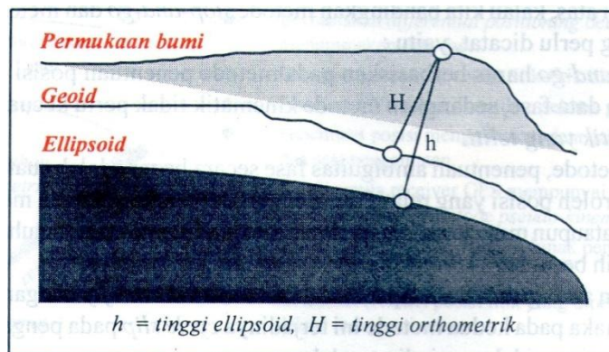
Gambar 4.19. Perbedaan tinggi ellipsoid dan Tinggi orthometrik
