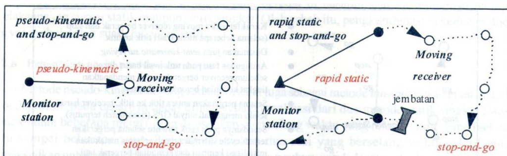
Gambar 4.18. Contoh kombinasi metode penentuan posisi
