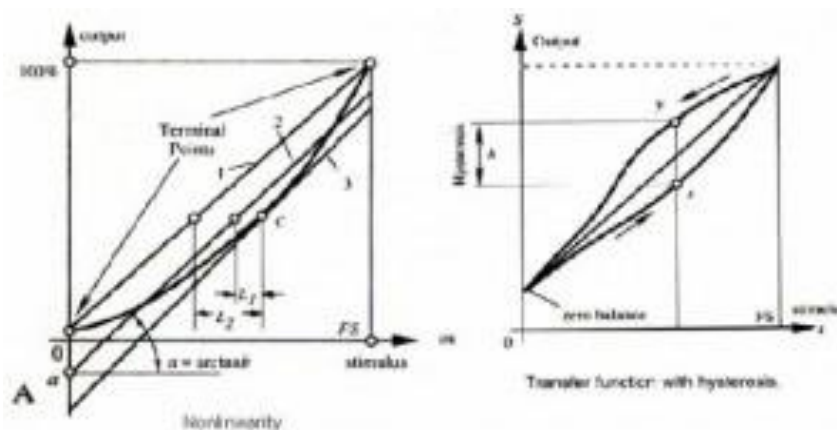
Gambar 5. Grafik Histeresis
