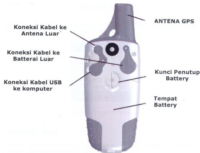
Gambar 5.2 Beberapa port yang ada di belakang
