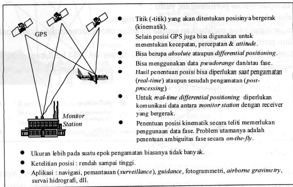
Gambar 4.13. Metode penentuan posisi kinematik
