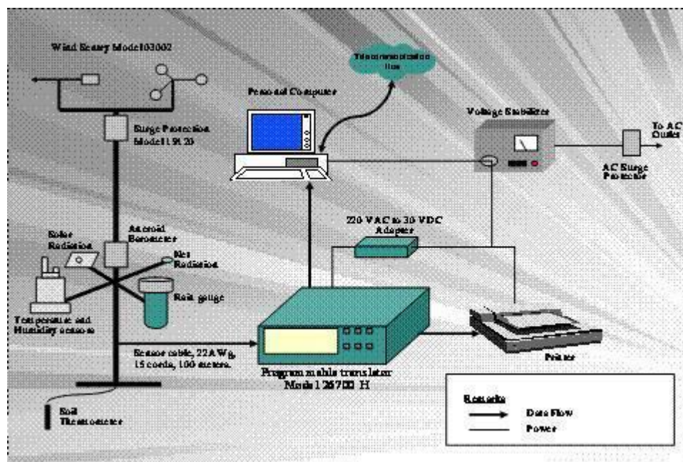
Gambar 2. Blok Diagram RM Joung AWS
