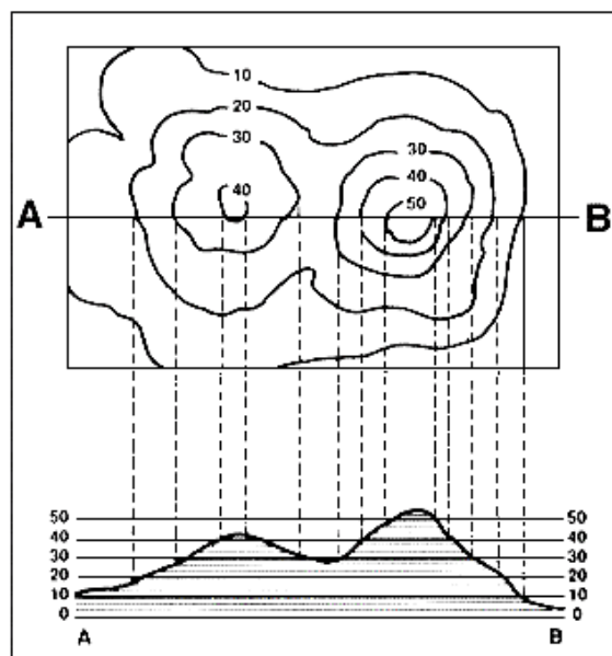
Gambar 6.1 Garis kontur dan penampangnya
