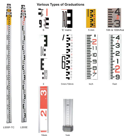
Gambar 2.3 Rambu ukur
