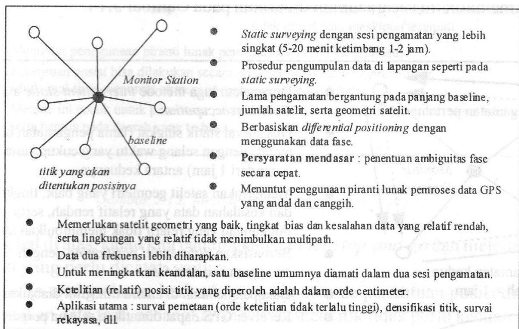
Gambar 4.14. Metode penentuan posisi secara statik singkat
