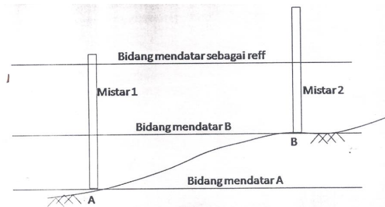
Gambar2.11. Beda tinggi A dan B
