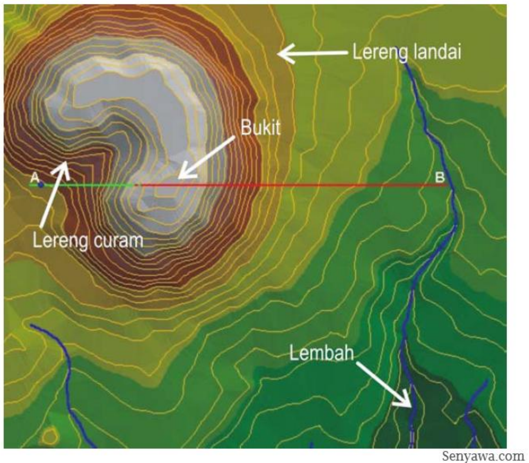
Gambar 6.2 Interpretasi bentuk lahan pada Peta Topografi
