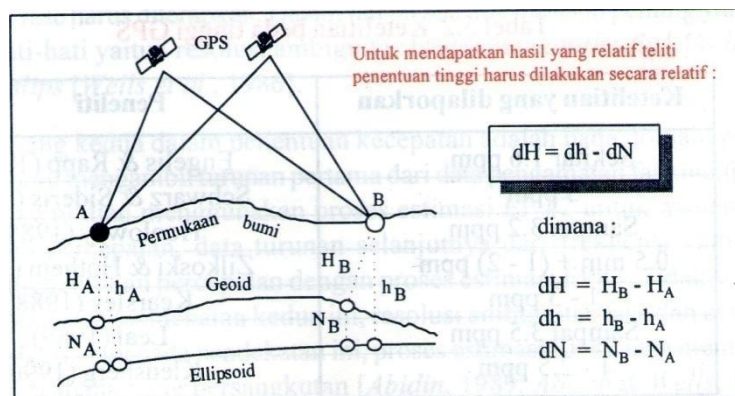
Gambar 4.21. Penentuan tinggi secara diferensial
