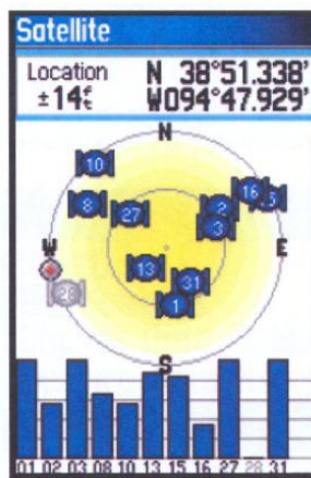
Gambar 5.3. Satelit page
