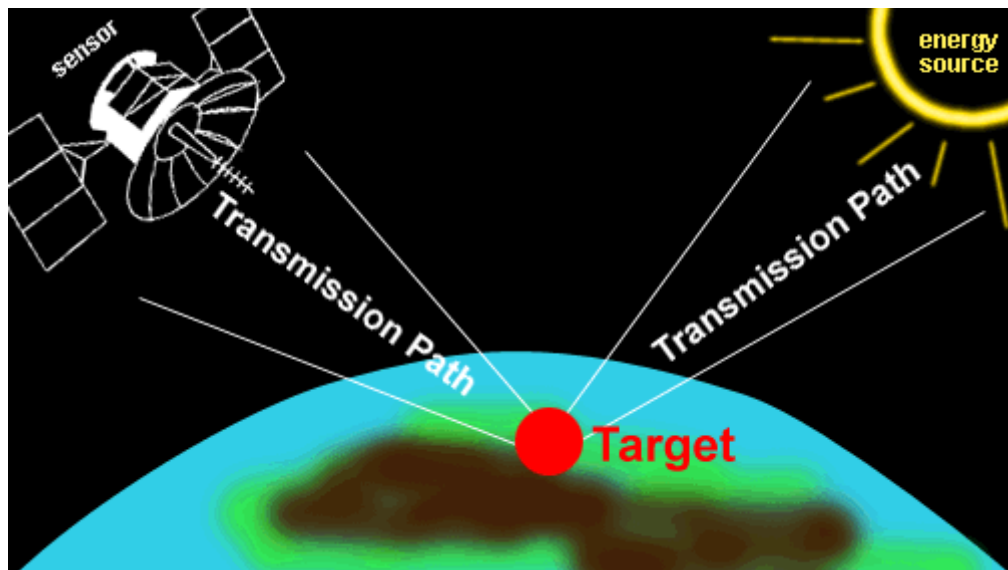
Gambar 7.2. Komponen Remote sensing ( Inderaja)
