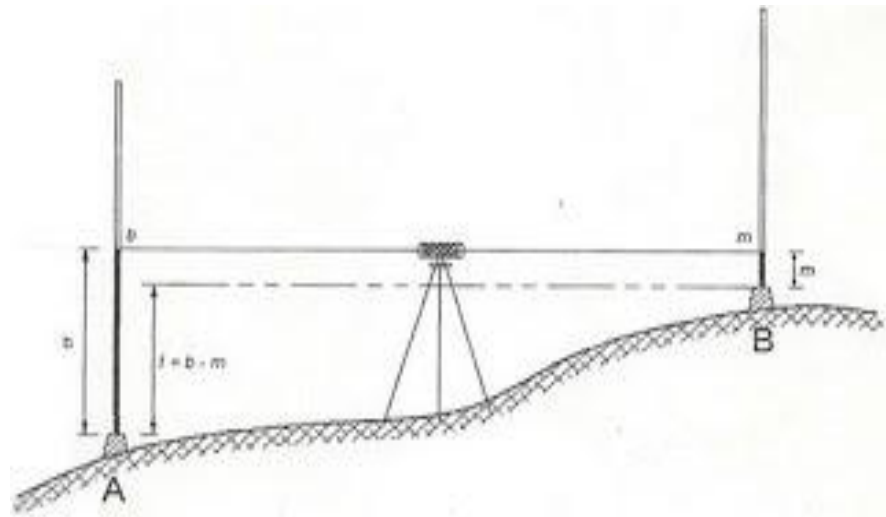
Gambar 2.12. Mengukur Beda tinggi dengan Sipat Datar
