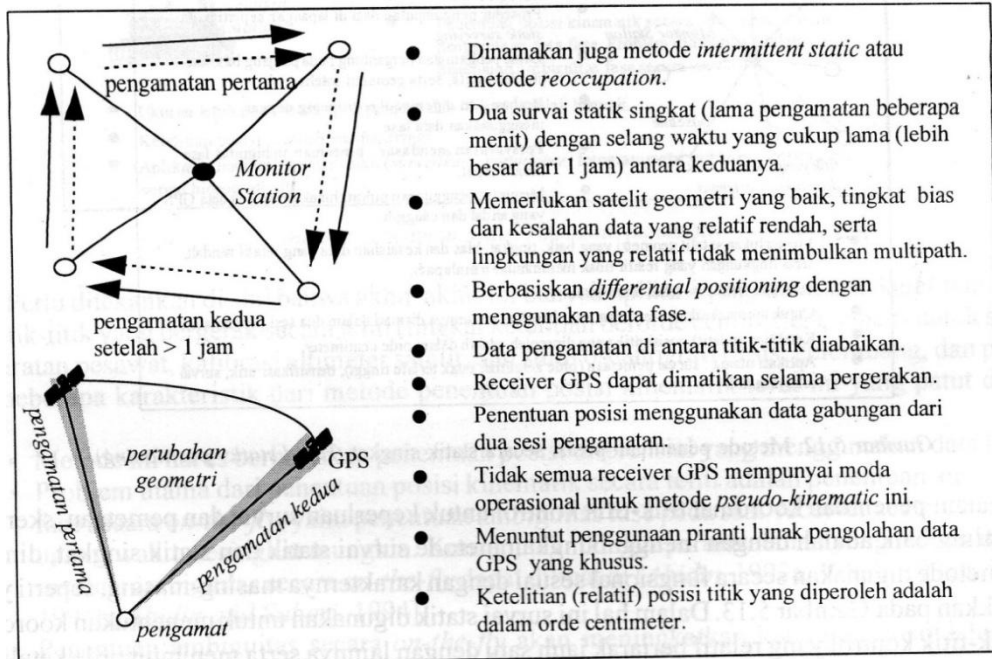
Gambar 4.16. Metode penentuan posisi pseudo-kinematik
