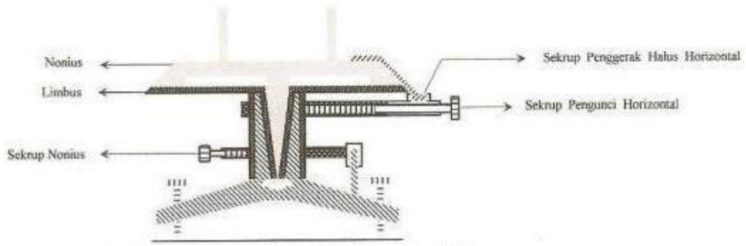
Gambar 3: Konstruksi Theodolite Type Repetisi
