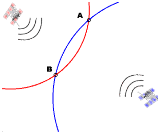
Gambar 4.6. Dengan dua range, receiver GPS bisa berada di kedua titik A atau titik B
