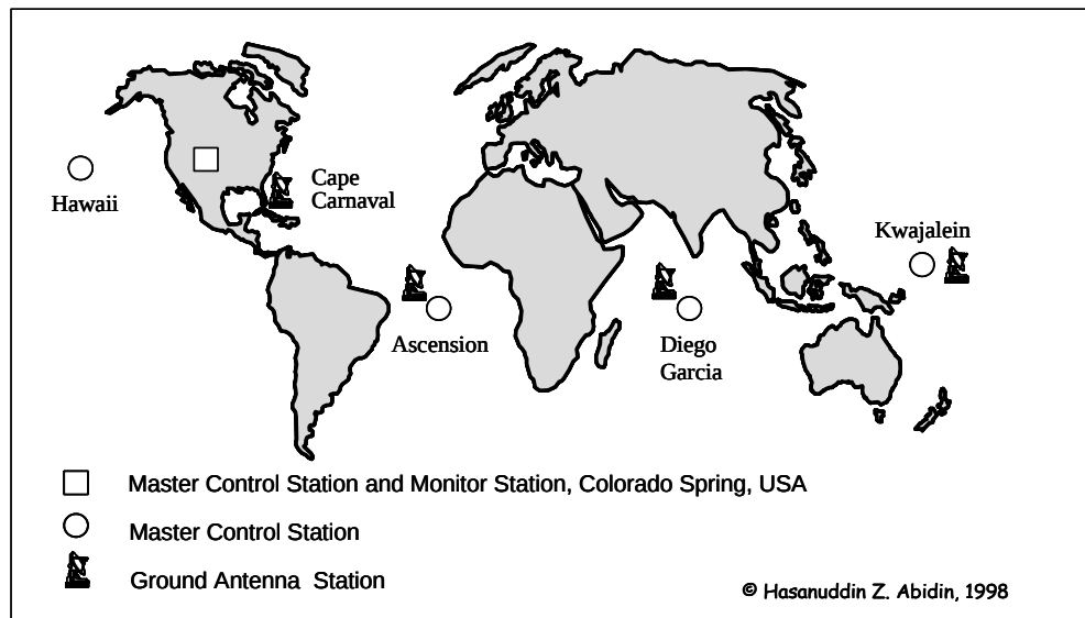
Gambar 4.3. Sistem Kontrol GPS
