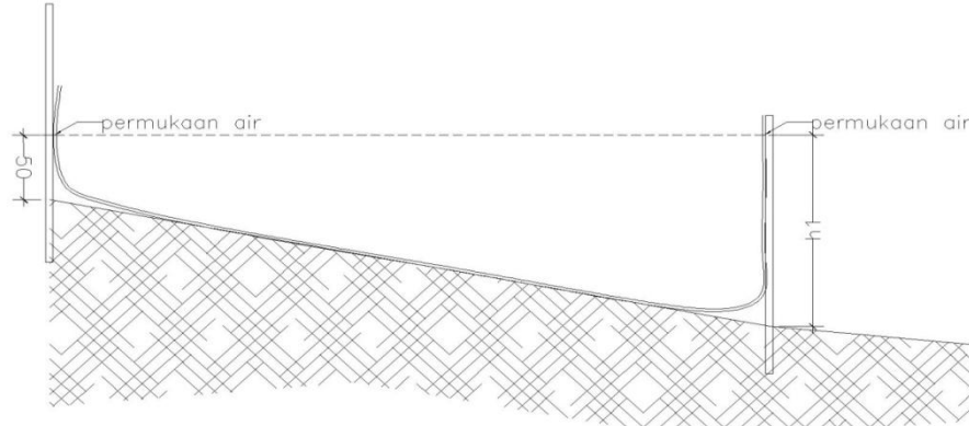
Gambar 2.9 Pengukuran beda tinggi dengan slang.
