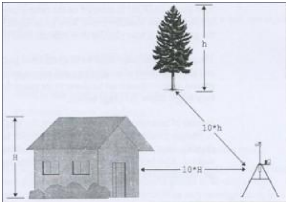
Gambar 3. Standarisasi Penempatan AWS
