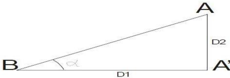
Gambar 6.23 . Perhitungan sudut miring lahan
