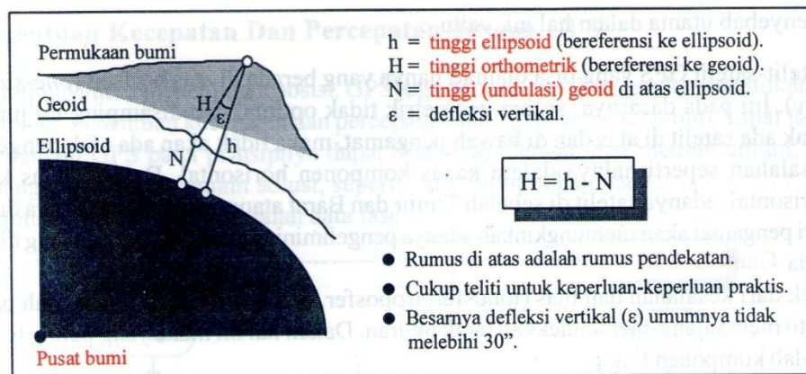
Gambar 4.20. Transformasi tinggi ellipsoid ke tinggi orthometrik
