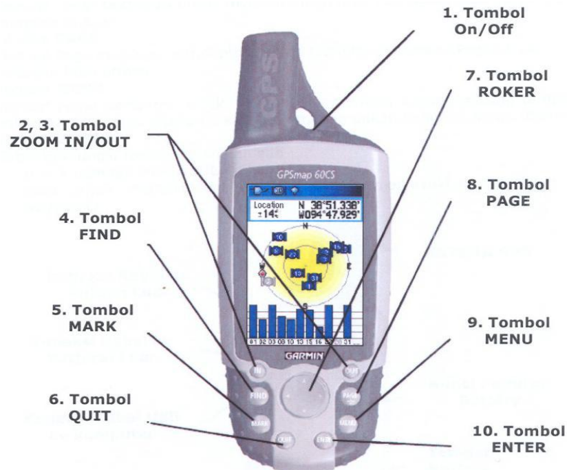
Gambar 5.1 Tombol utama garmin Map 60 CSX
