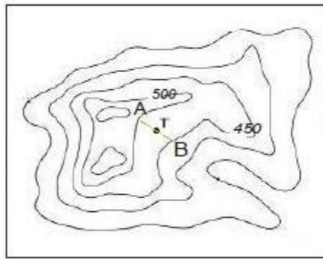
Gambar 6.22. Contoh mencari tinggi titik dengan kontur
