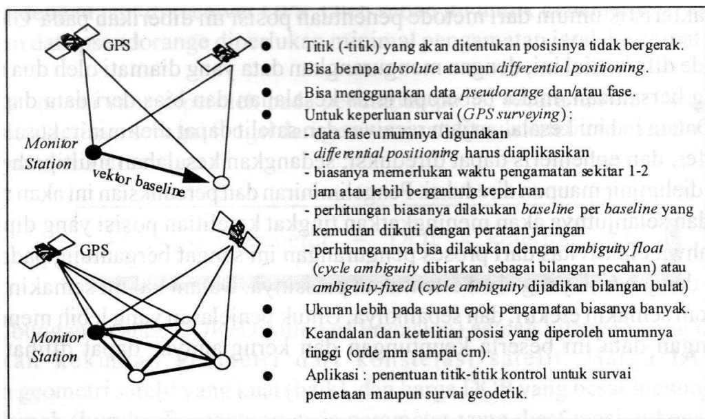
Gambar 3.12. Penentuan posisi titik-titik dengan metode survey GPS
