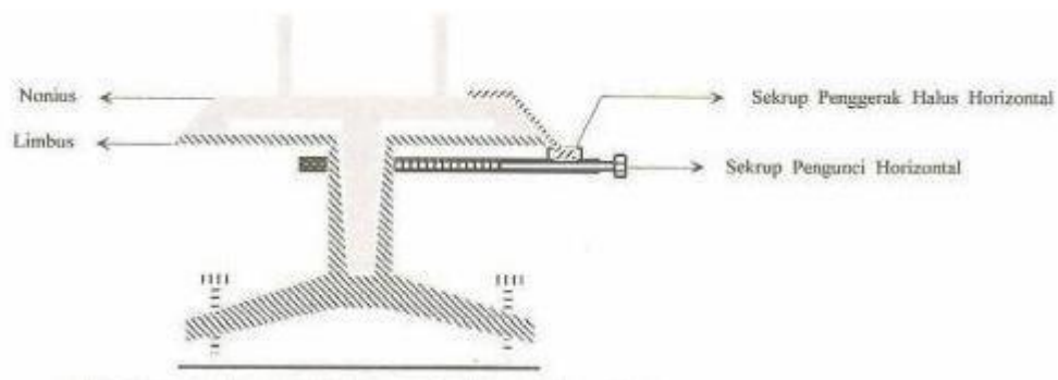
Gambar 2: Konstruksi Theodolite Type Reiterasi
