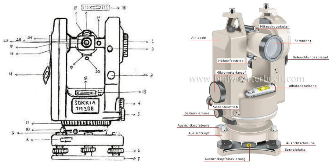
Gambar 5: Sketsa Theodolite SOKKIA TM20E pandangan dari belakang
