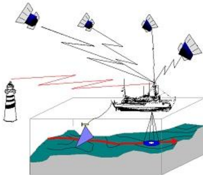
Gambar 1.2 Survei Hidrografi
