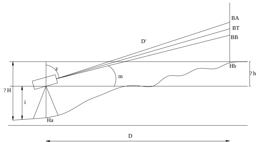
Gambar 2.2. Pengukuran cara Trigonometrik
