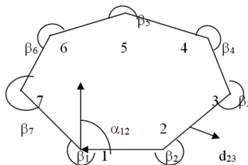
Gambar 3.8. Poligon tertutup
