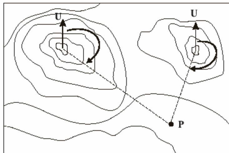
Gambar 6.20. Koordinat titik menggunakan arah dan arah
