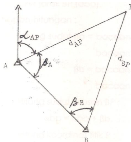
Gambar 3.2 Metoda perpotongan ke muka
