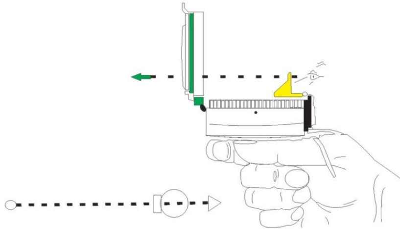
Gambar 2.3 Cara menggunakan kompas dengan benar
