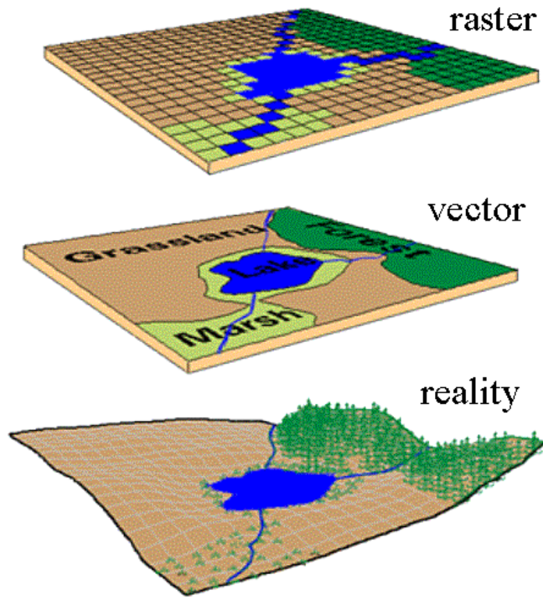
Gambar 7.5. Ilustrasi Data raster dan data vector yang selanjutnya ditampilkan dalam dunia nyata
