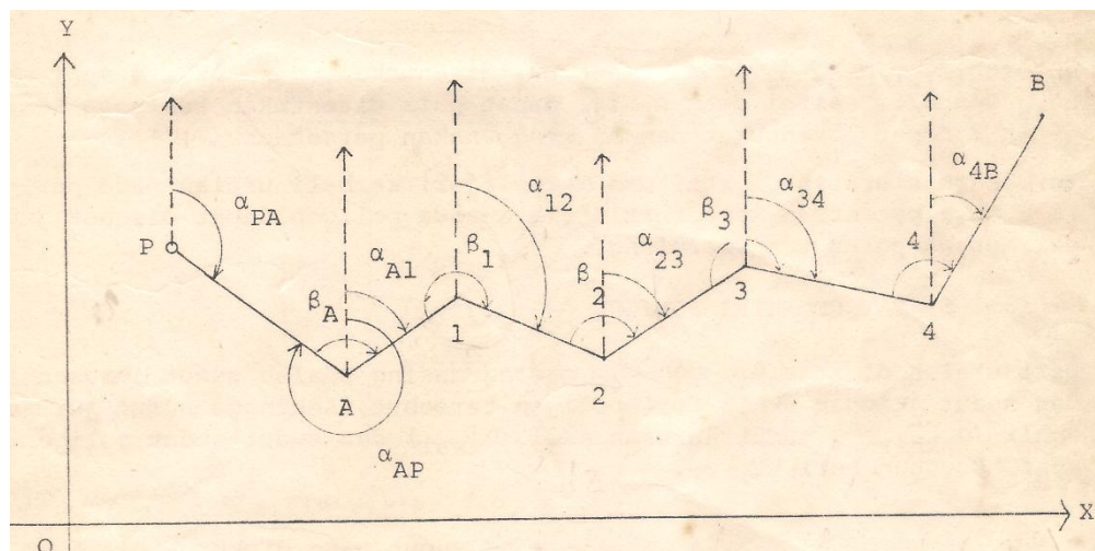
Gambar 3.7. Prinsip dasar Hitungan Sudut Jurusan Sisi Poligon
