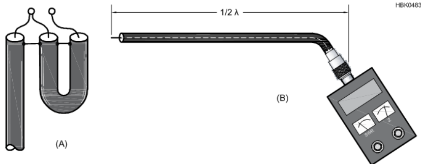
Gambar 3.2. Cara membuat balun
