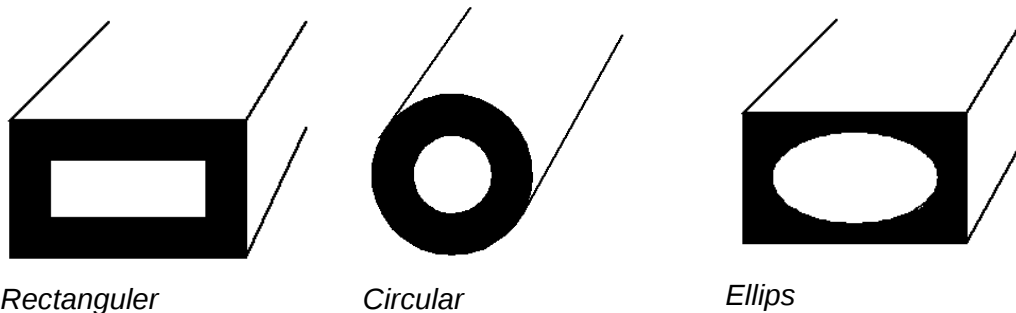
Gambar 5.1. Jenis waveguide
