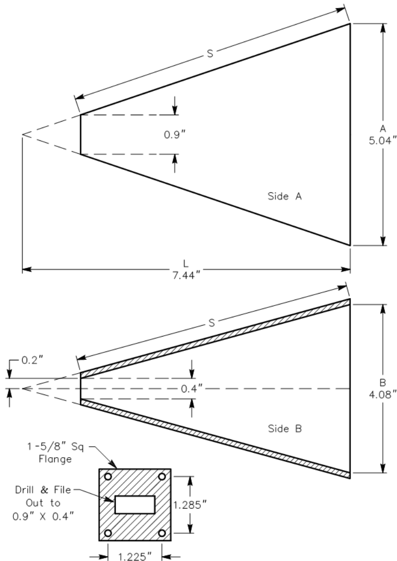
Gambar 4.4. Dimensi potongan antenna corong 10GHz.
