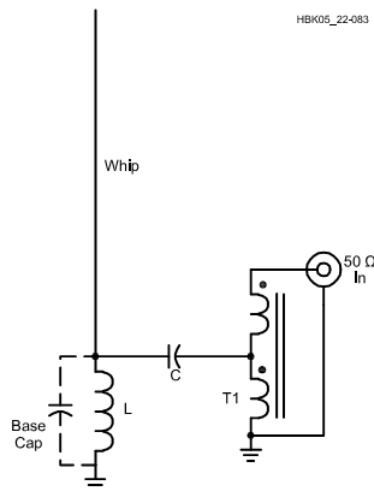
Gambar 1.5. Rancangan antenna mobil HF
