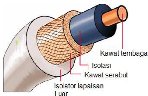
Gambar 9.1 Kabel koaksial
