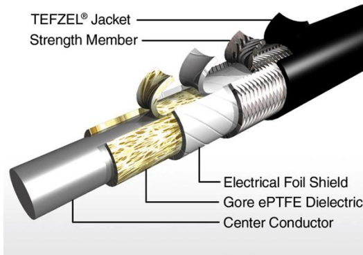
Gambar 8.2 Kabel PTFE
