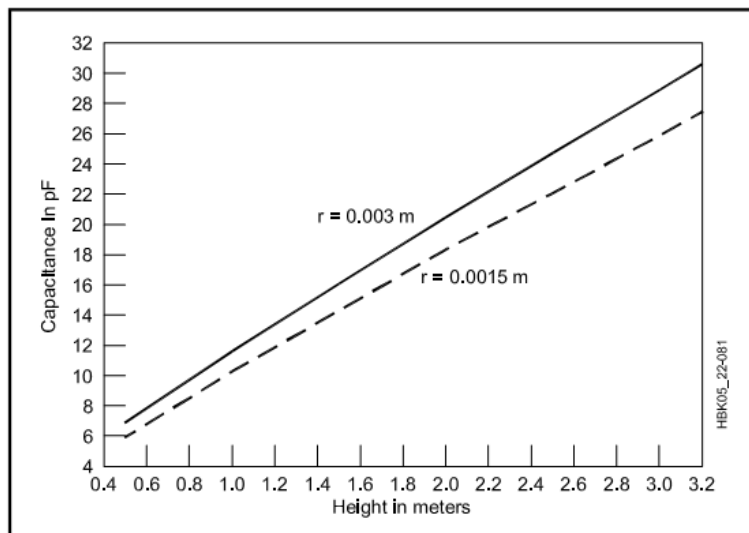
Gambar 1.1. Grafik penambahan kapasitor terhadap tinggi antenna di frekuensi 3,5MHz
