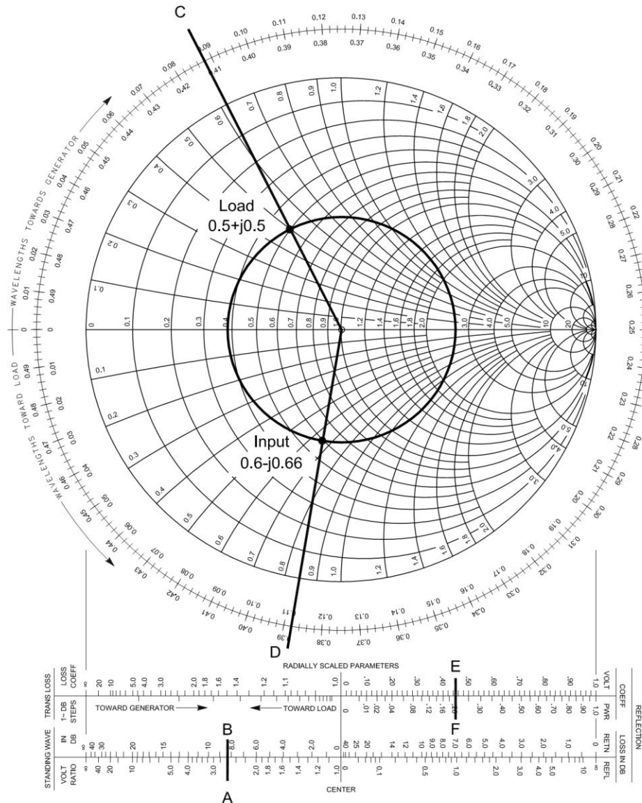
Gambar 6.6. Hubungan antara Input dan beban
