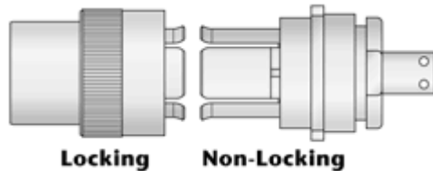
Gambar 10.16. Konektor GR874
