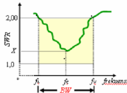
Gambar 5.11. Bandwidth pada antenna
