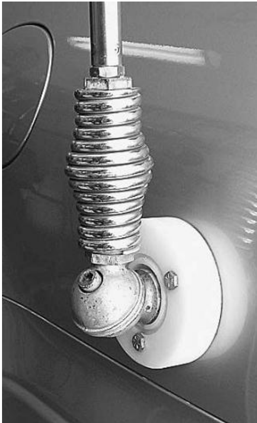
Gambar 1.8. Salah stu contoh pemasangan antenna mobil HF di kendaraan
