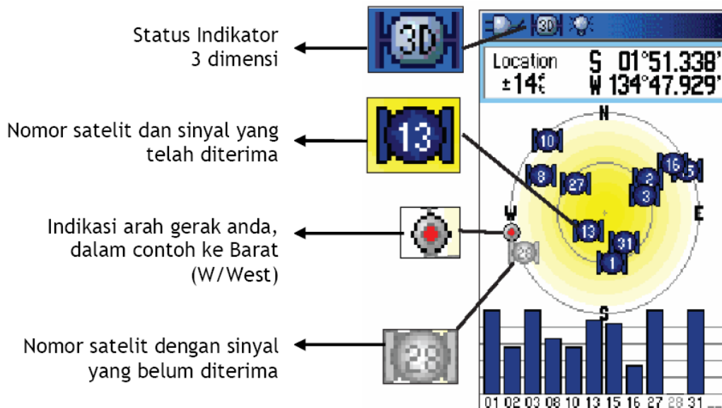
Gambar 7. Fungsi dan keterangan tombol pada contoh GPS yang ada di pasaran
