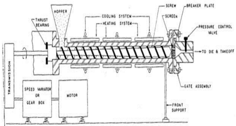
Gambar 31. Prinsip kerja extruder
