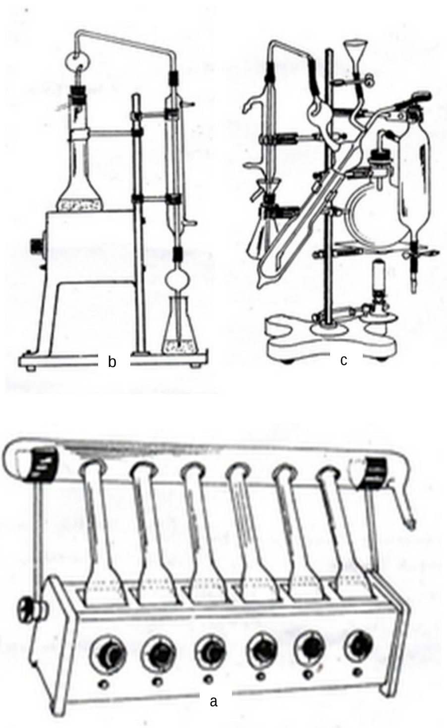
Gambar 39 : (a). Pendidihan (destruksi) bahan dalam labu Kjeldahl; (b). Alat destilasi; (c). Alat dstilasi mikro Kjeldahl
