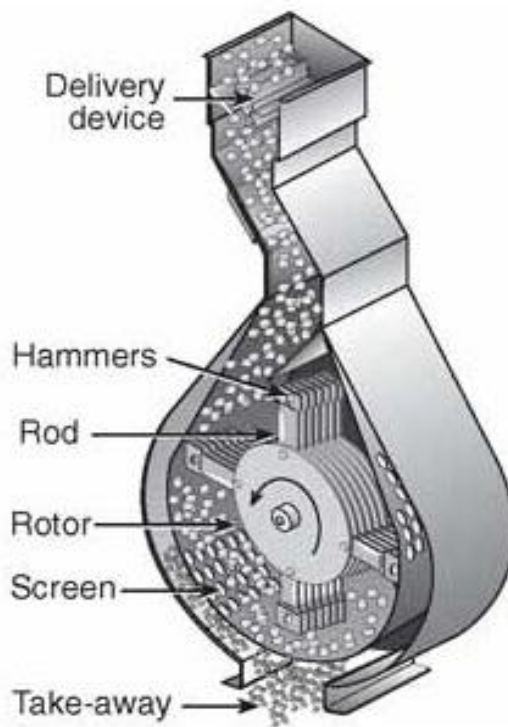
Gambar 16. Bagian – bagian hammer mill
