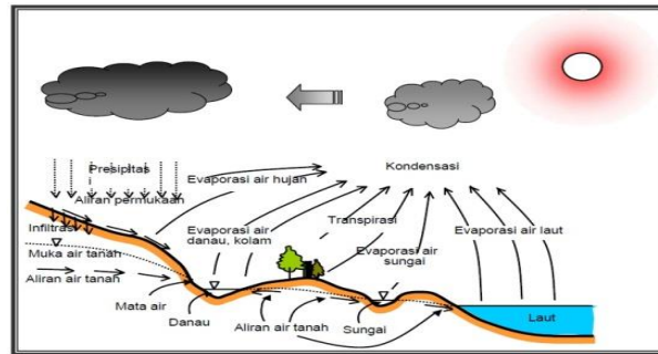
Gambar 8. siklus air
