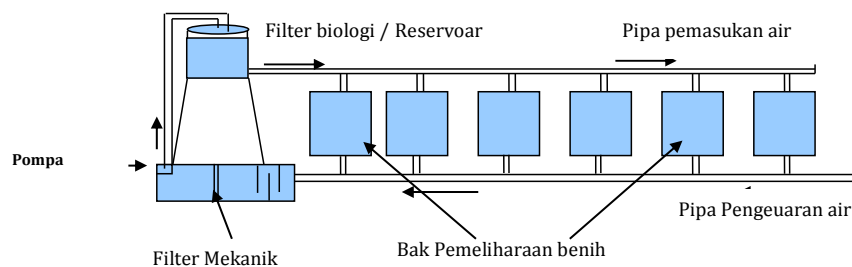
Gambar 88. Resirkulasi Air
