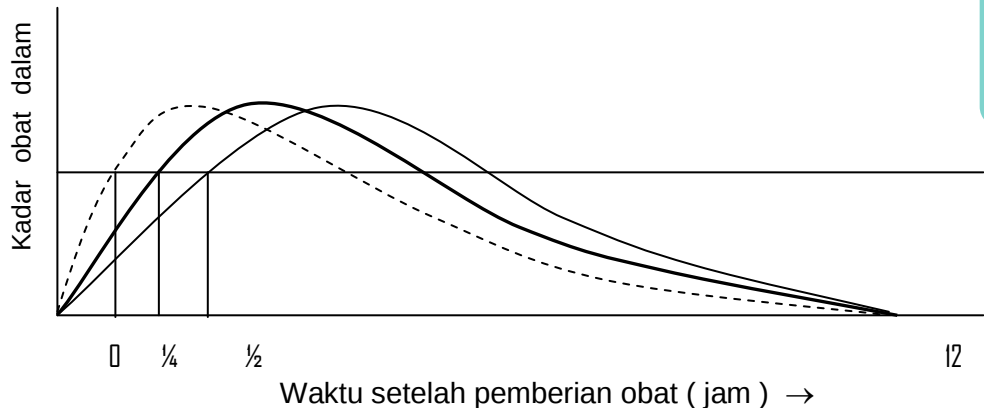
Grafik 1.1. kadar obat dalam darah versus waktu setelah pemberian obat
