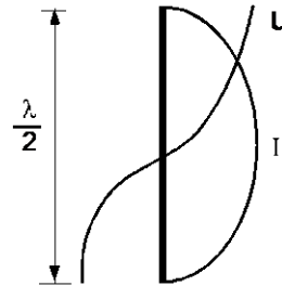
Antena dipol
