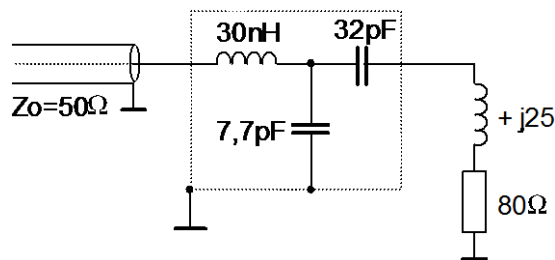
Gambar 6.3. Rangkaian penyesuai LC ( R_a > Z_0 )
