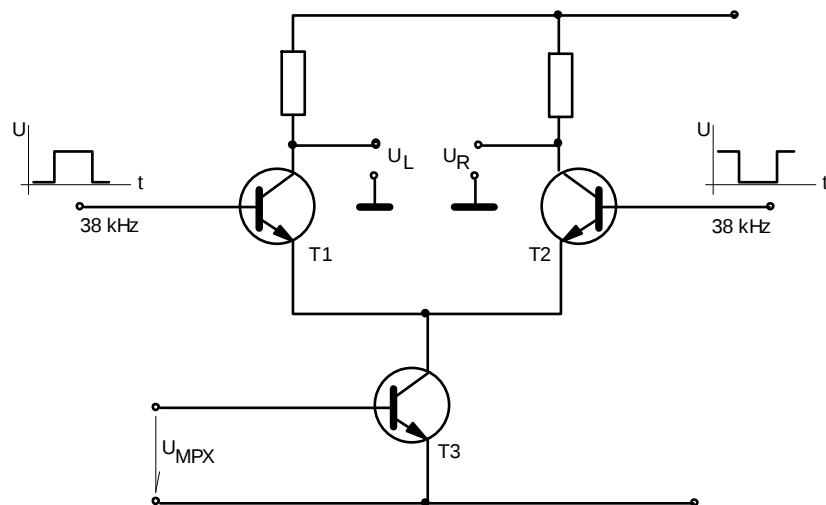
Gambar 17.16 Saklar elektronika
