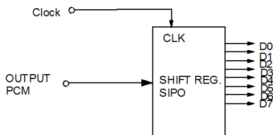
Gb.20.1 Shift register SIPO
