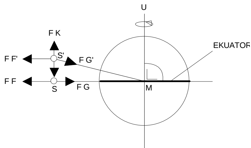
Gambar 7.4 Ekuator
