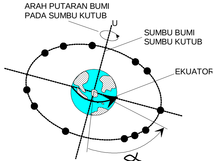
Gambar 7.3 Peredaran satelit
