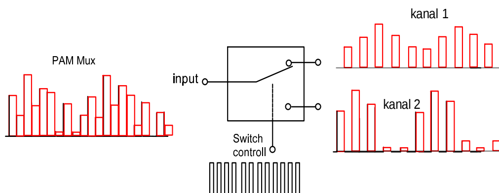
Gambar 20.7 De-multiplexing 2 kanal
