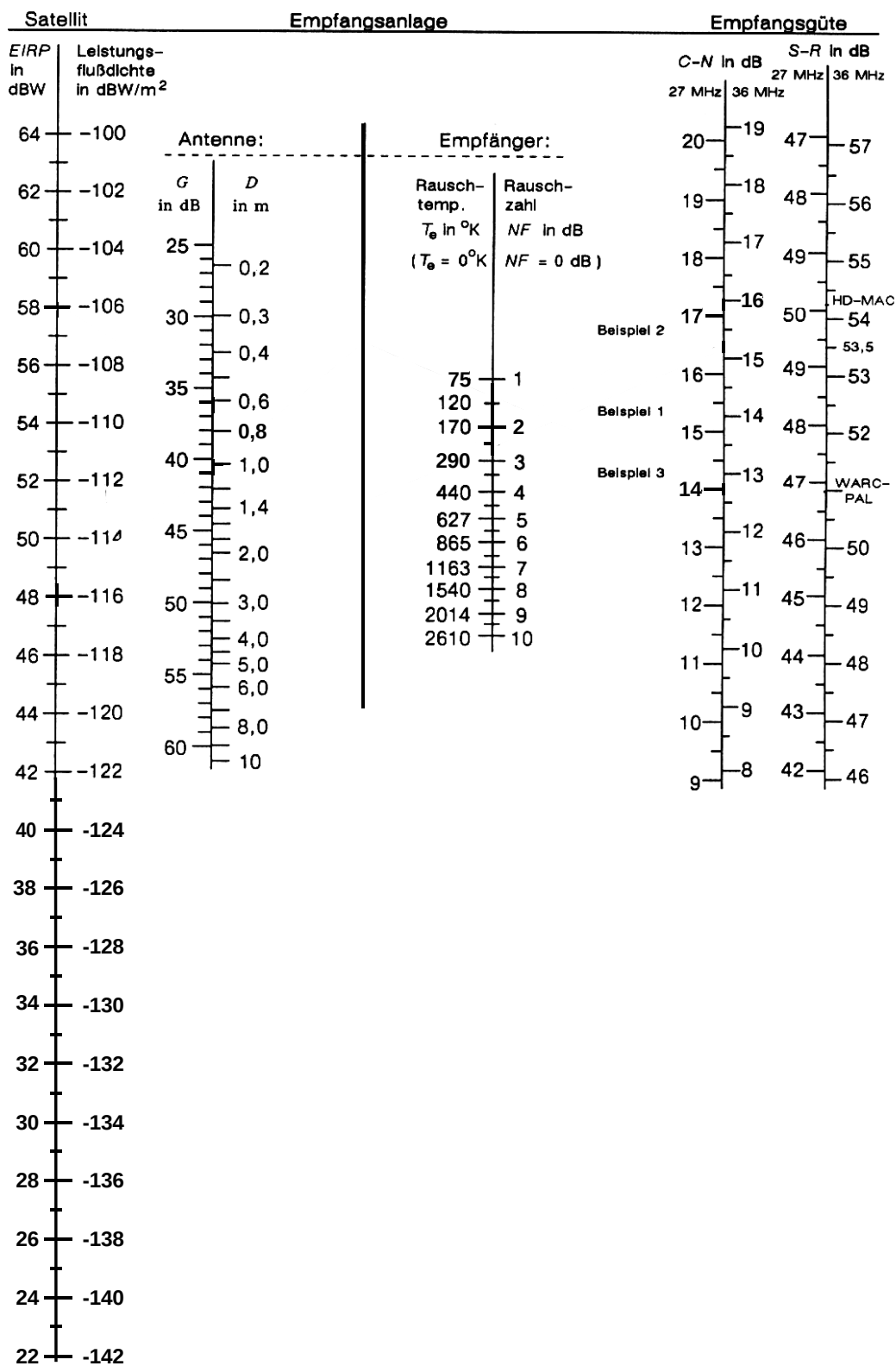
Gambar 10.1 Nomogram untuk perhitungan pesawat penerima
