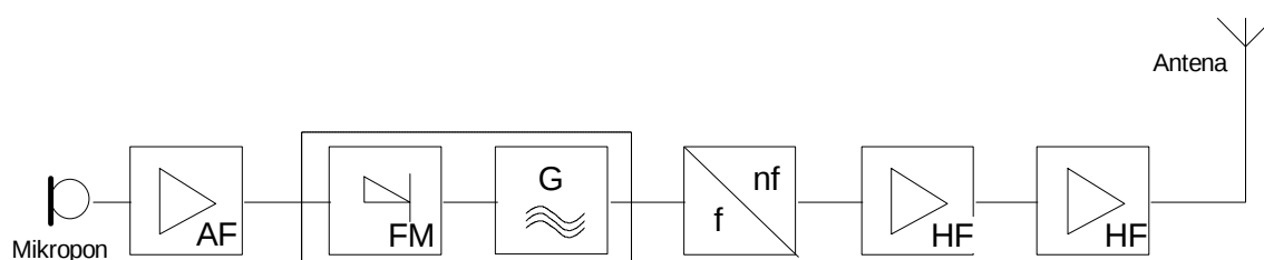
Gambar 14.2 Blok pemancar FM
