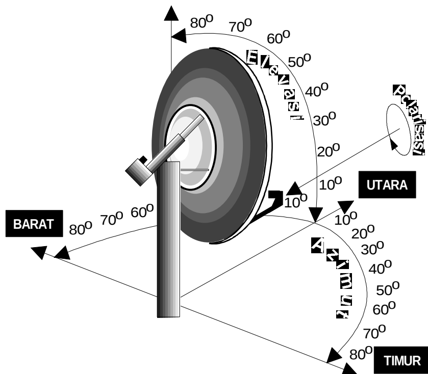
Gambar 7.12 Sudut pengaturan pada pengarahannya metoda azimut elevasi.
