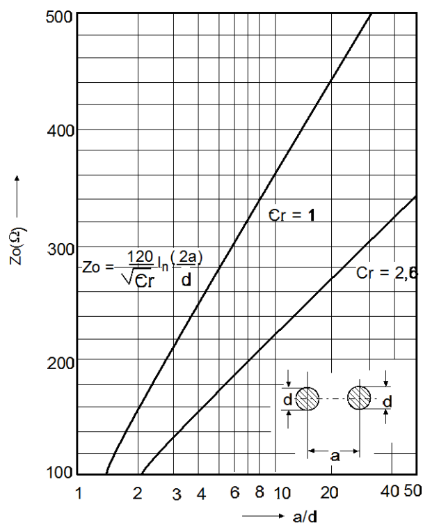
Gambar 5.8 Tahanan gelombang
