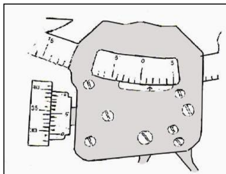
Gambar 75. Sextan tromol dengan pembacaan positif
