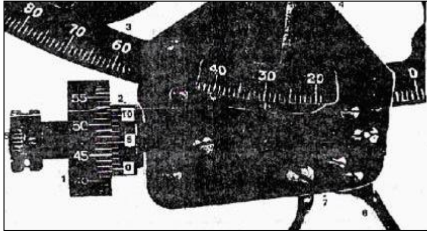
Gambar 74. Sextan tromol dengan pembacaan positif
