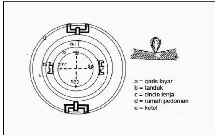
Gambar 65. Cincin Lenja
