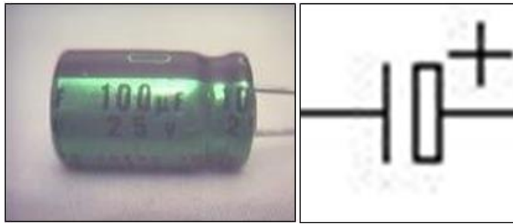
Gambar 20. Lambang Kapasitor Mempunyai Kutub Negatif dan Positif Pada Skema Elektronika
