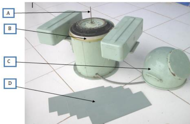
Gambar 77. Kompas Baring dan Perlengkapannya
