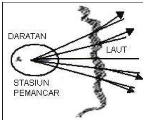
Gambar 92. Pengaruh Pantai
