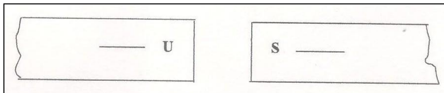
Gambar 5. Muatan Berbeda Tarik Menarik
