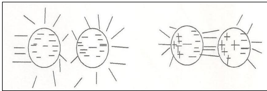
Gambar 7. Kutub Sejenis (kiri) dan kutub tidak Sejenis (kanan)
