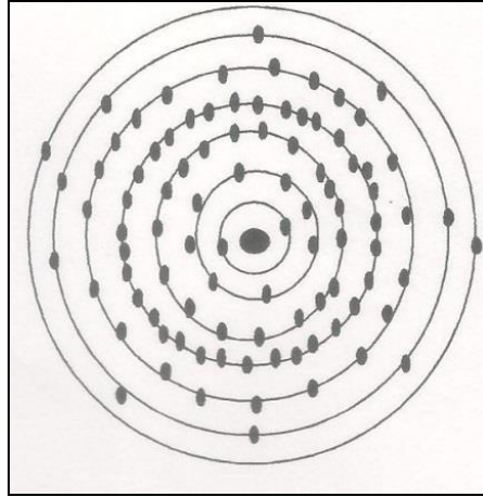
Gambar 2. Atom Uranium
