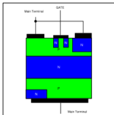
Gambar 35. Kontruksi Simbol TRIAC
