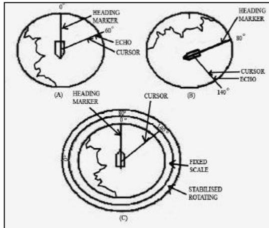
Gambar 98. Penentuan posisi dengan Radar
