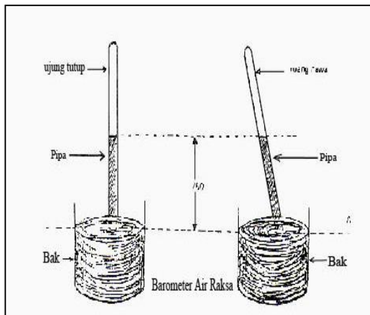
Gambar 80. Barometer Air Raksa
