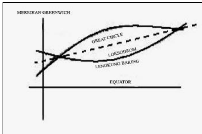
Gambar 93. Bentuk gambar lingkaran besar, loksodrom, lengkungan baring pada peta Mercator
