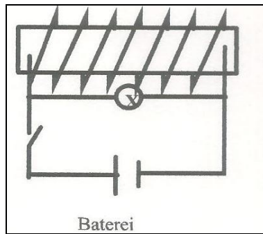
Gambar 12. Induksi sendiri
