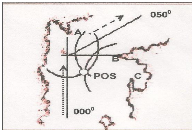
Gambar 103. Pengukuran Jarak Tiga Benda
