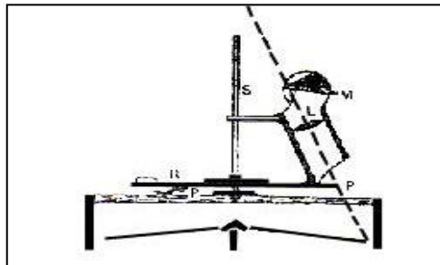
Gambar 79. Pesawat Baring Thomson
