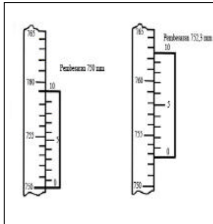
Gambar 81. Nonius
