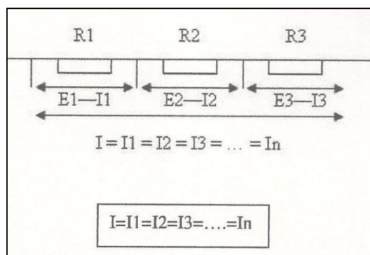
Gambar 19. Resistor Seri atau Deret
