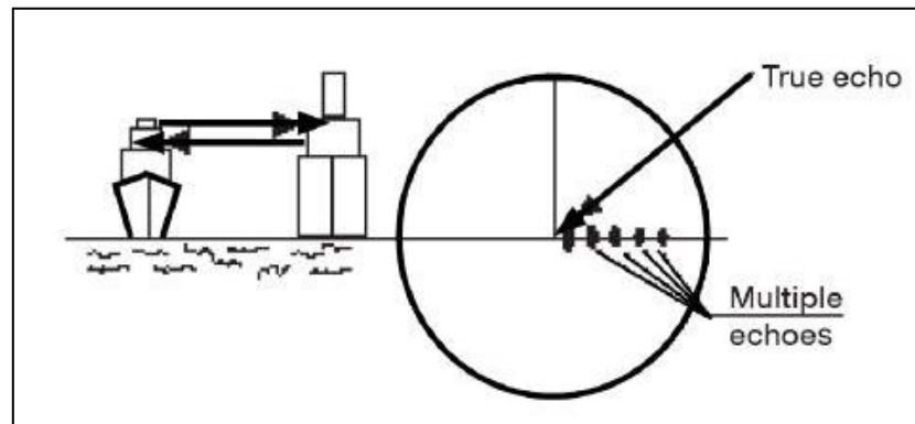
Gambar 105 Multi Gema melebihi gema target asli
