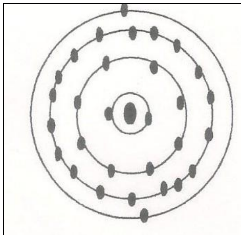
Gambar 3. Atom Tembaga
