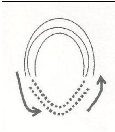
Gambar 6. Besi magnet berbentuk tapak kuda dengan sebagian garis gayanya.
