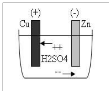
Gambar 24. Ion ion Elektron
