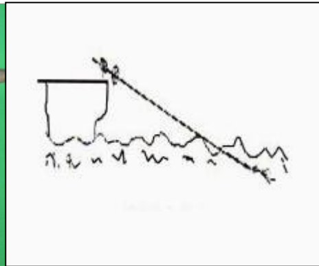
Gambar 55. Aria Topdal
