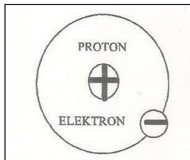
Gambar 1. Atom Hidrogen
