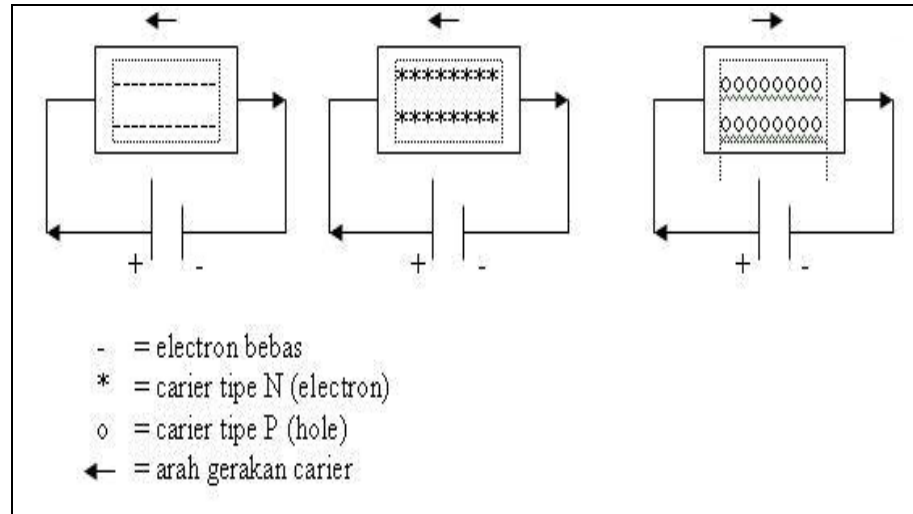
Gambar 26. Elektron bebas
