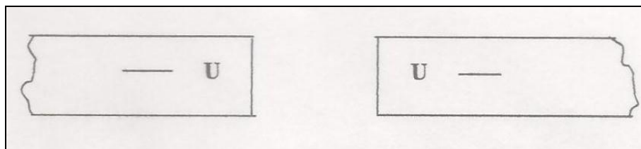
Gambar 4. Muatan yang sama tolak menolak
