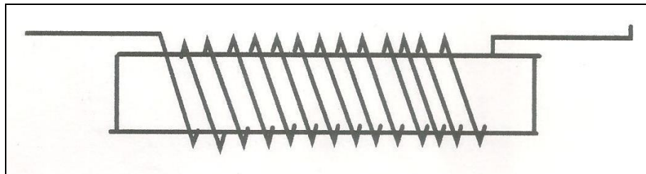
Gambar 11. Penghantar dalam beberapa gulungan akan memperkuat medan magnet.
