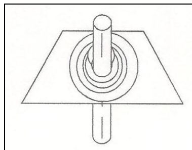
Gambar 8. Bentuk medan magnet di sekeliling penghantar
