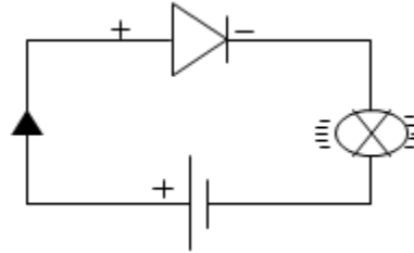
Gambar 27. Cara Pemasangan Dioda
