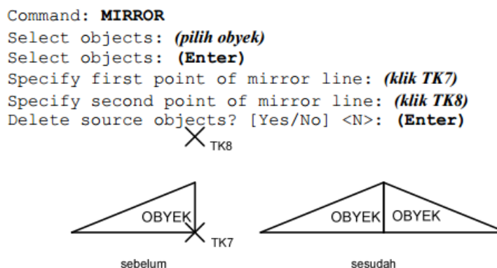
Gambar 6.4. Pencerminan MIRRTEXT=0
