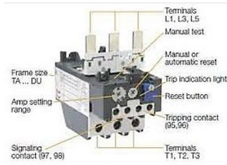
Gambar 1.3 Kontruksi dan TOL / Thermal Over load ( Beban Lebih )
