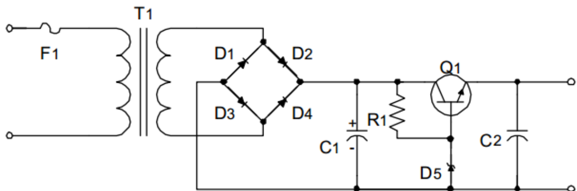
Gambar 1.5 rangkaian penyearah dengan stabilisator tegangan
