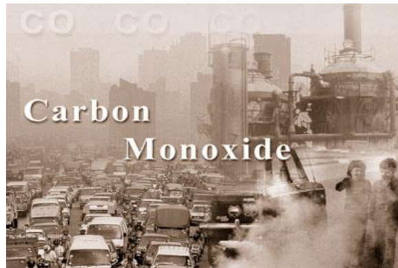
Gambar 5. Gas karbon monooksida hasil pembakaran kerndaraan bermotor (sumber: google.com)
