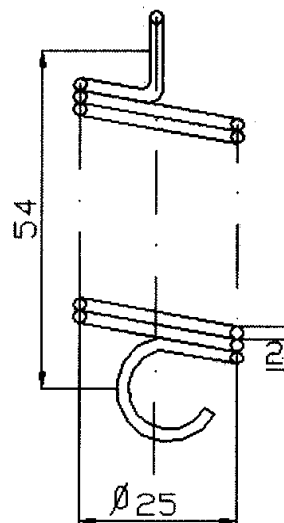
Gambar 3. 83 Pegas
