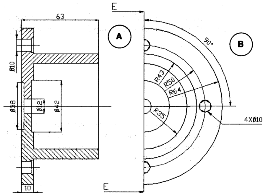
Gambar 3. 102 Dudukan baut
