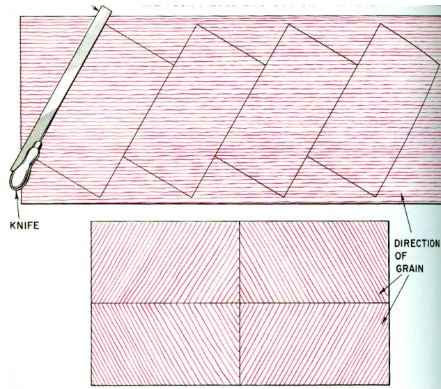
Gambar 7. Cara melukis bentuk dan ukuran vinir yang akan dipotong
