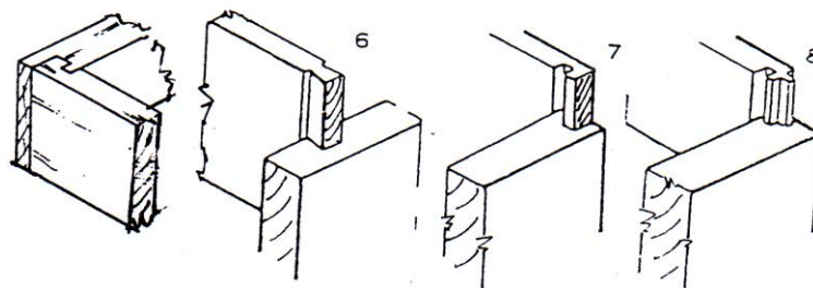
Gambar Detail Konstruksi Hubungan Laci
