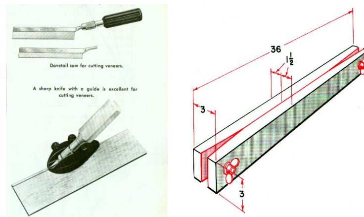
Gambar 6. Gergaji vinir dan Penggapit Vinir
