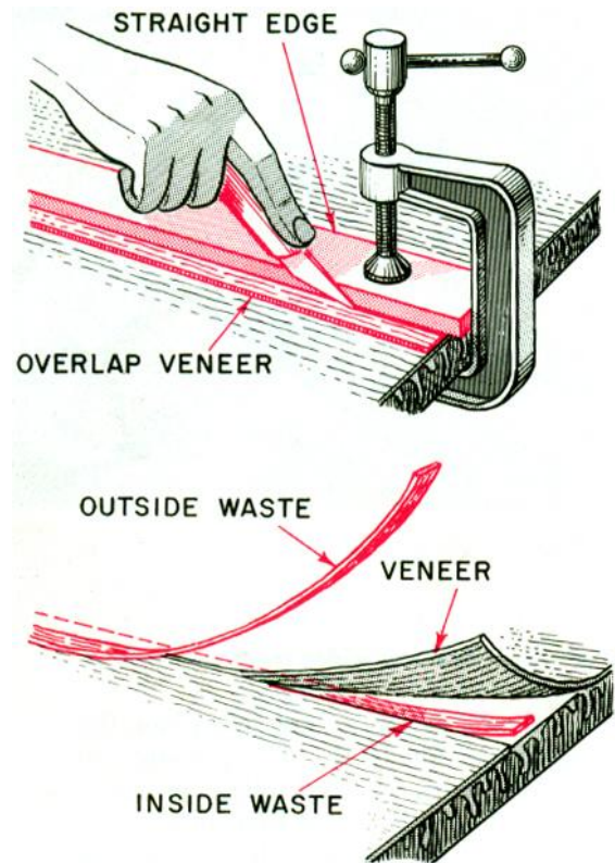
Gambar 16. Memotong vinir
