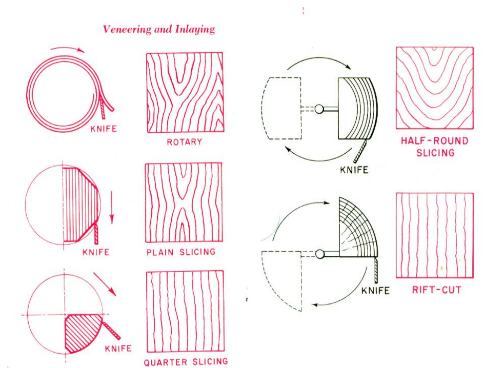
Gambar 5. Pembuatan Vinir pada Proses Rotary dan Slicing
