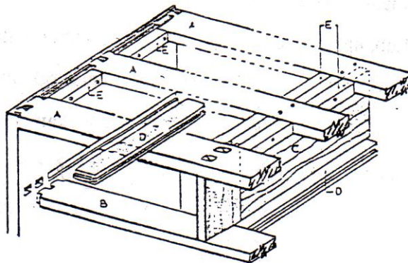
Gambar.. Rangka Tempat Dudukan Laci
