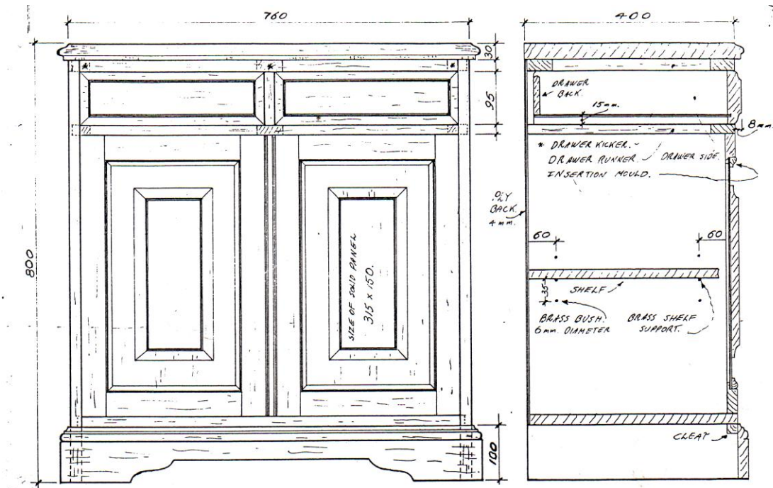
Gambar Konstruksi Panel Solid
