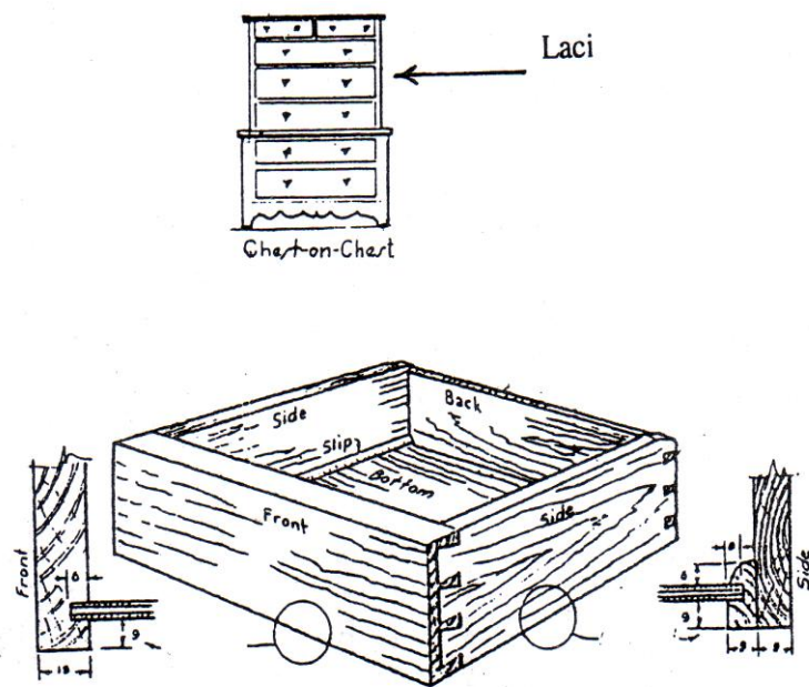
Gambar. Konstruksi Laci dan Pemasangannya
