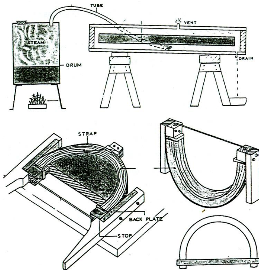
Gambar 15. Peralatan untuk Pekerjaan Steam Bending
