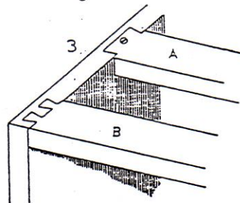
Konstruksi dengan Ekor burung tunggal/ganda
