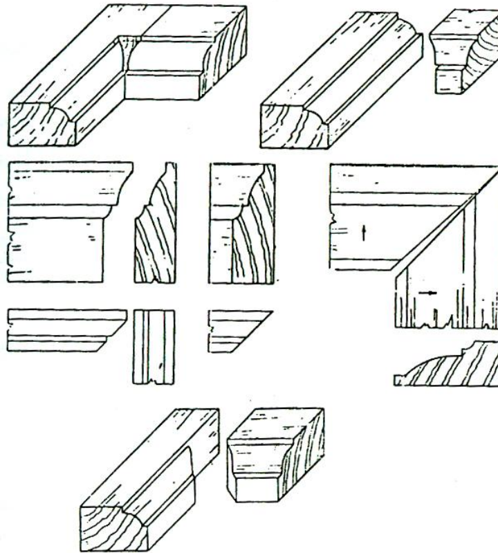
Gambar 12. Pemasangan Profil
