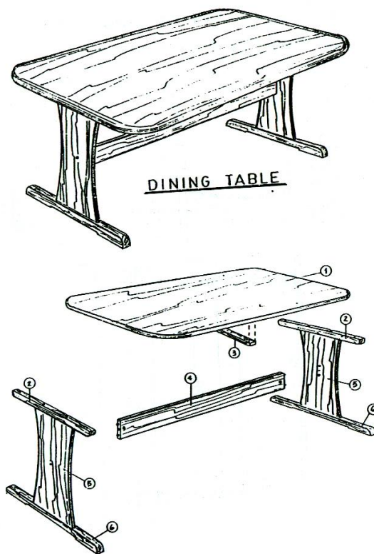
Gambar. Tipikal Konstruksi Meja Sederhana
