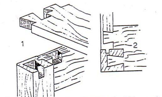
Konstruksi dengan Ekor burung dada tidak segaris
