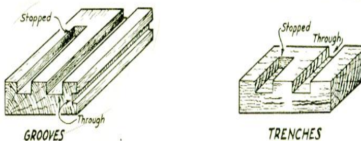
Gambar 3. Grooved / Alur tembus dan Buntu & Trenches
