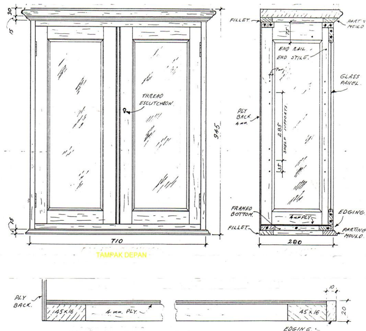
Gambar Aplikasi Konstruksi Rangka Datar
