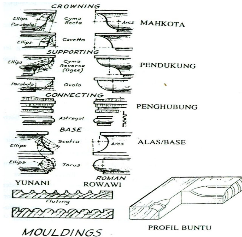
Gambar 10. Kelompok Moulding dan Profil
