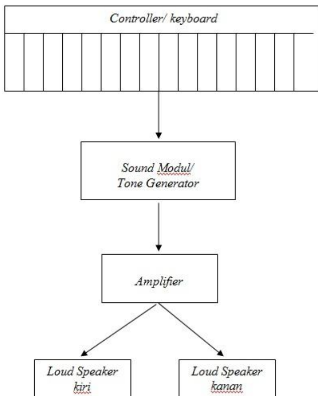
Gambar 160: Susunan peralatan pada keyboard
