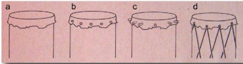
Gambar 109: Berbagai pemasangan membran, dengan:
