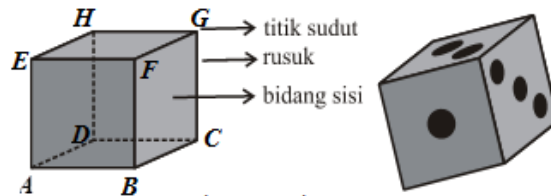
Gambar 59. Kubus
