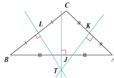
Gambar 17. Garis Sumbu Segitiga
