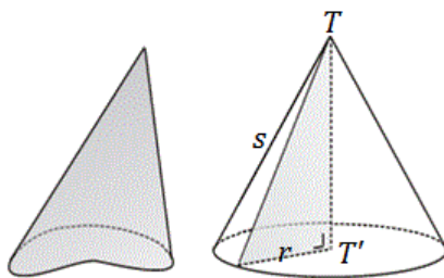
Gambar 78. Kerucut
