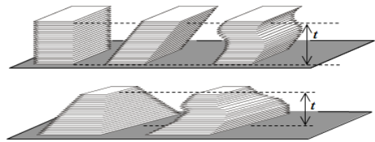
Gambar 69. Prinsip Cavalieri
