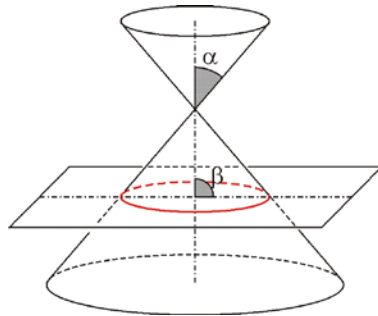
Gambar 95. Irisan kerucut dan bidang berupa lingkaran
