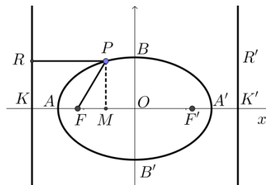
Gambar 106. Ellips dengan pusat O(0,0)
