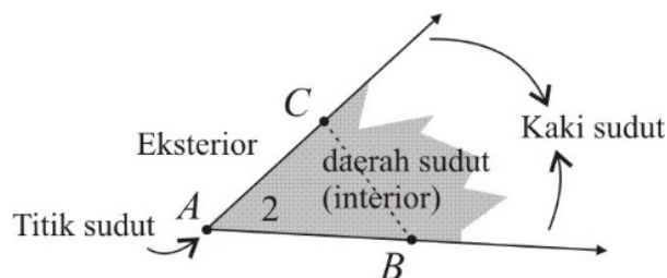
Gambar 3. Sudut
