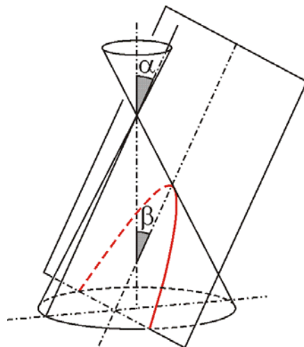
Gambar 97. Irisan kerucut dan bidang berupa parabola
