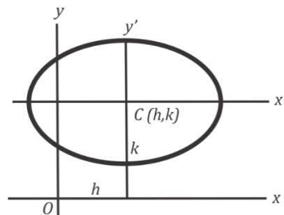
Gambar 108. Ellips berpusat di (h, k)
