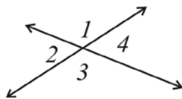
Gambar 7. Sudut bertolak belakang
