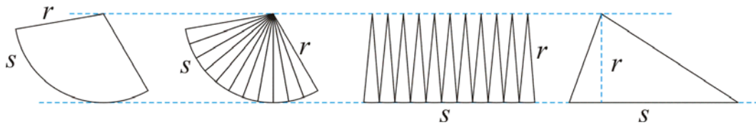
Gambar 79. Luas Selimut Kerucut
