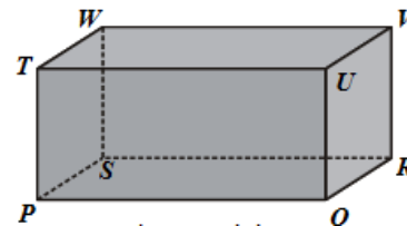
Gambar 60. Balok
