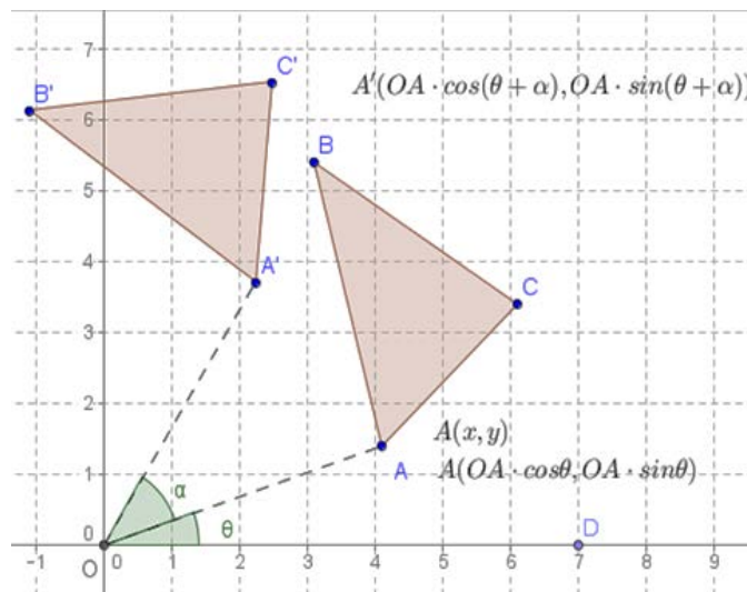
Gambar 44. Rotasi berpusat di (0, 0)
