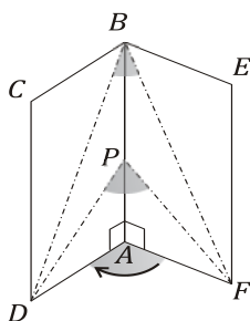
Gambar 92. Sudut antara Bidang dan Bidang
