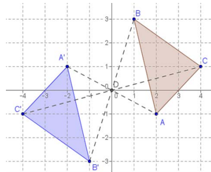
Gambar 55. Refleksi Terhadap Titik O
