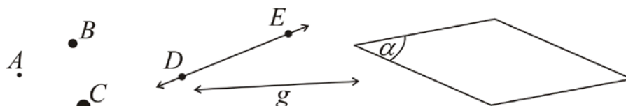
Gambar 1. Titik, Garis, dan Bidang
