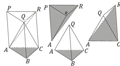
Gambar 73. Volume Limas Segitiga
