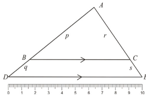
Gambar 22. Proporsi
