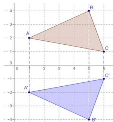
Gambar 50. Refleksi terhadap Sumbu- x
