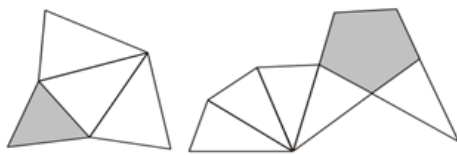
Gambar 75. Jaring-jaring Limas
