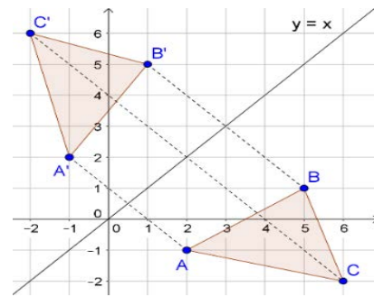
Gambar 52. Refleksi y = x
