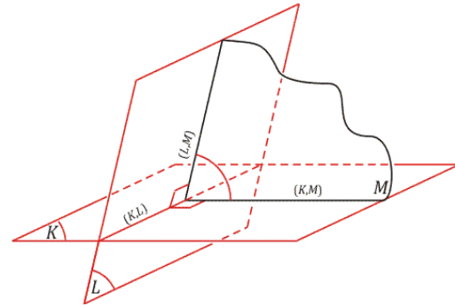
Gambar 93. Bidang Tumpuan
