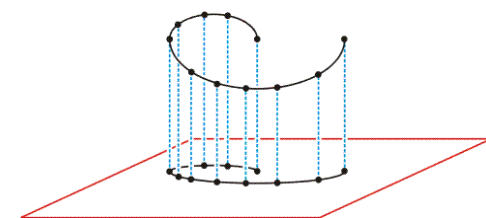
Gambar 85. Proyeksi Kurva ke Bidang
