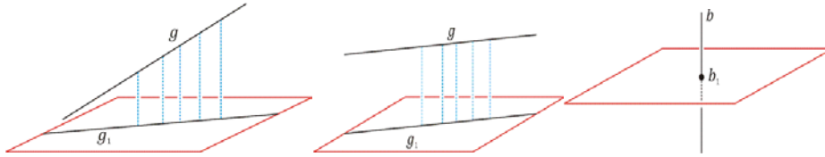
Gambar 86. Proyeksi Garis ke Bidang
