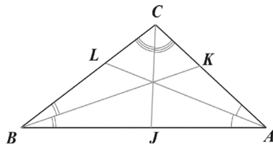
Gambar 20. Garis Bagi Sudut Segitiga
