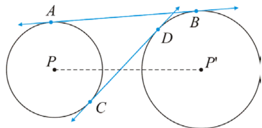
Gambar 40. Garis Singgung Persekutuan
