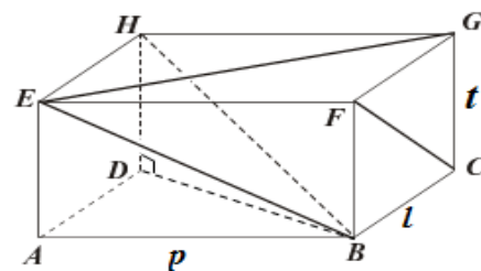
Gambar 64. Diagonal Sisi dan Diagonal Ruang
