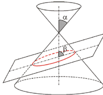
Gambar 96. Irisan kerucut dan bidang berupa ellips
