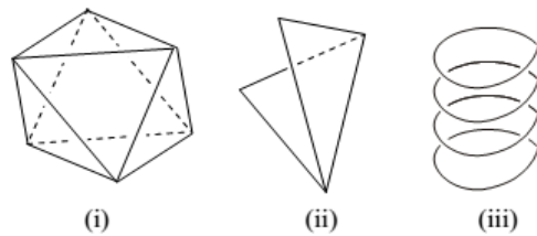
Gambar 58. Obyek berdimensi tiga
