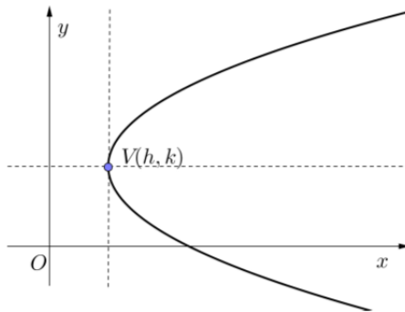
Gambar 104. Parabola yang puncaknya di V(h, k)
