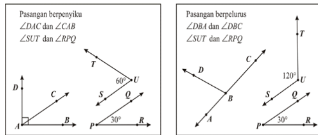
Gambar 6. Sudut Berpenyiku dan Berpelurus
