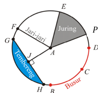
Gambar 34. Lingkaran dan bagian-bagiannya
