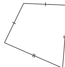
Gambar 32. Layang-layang
