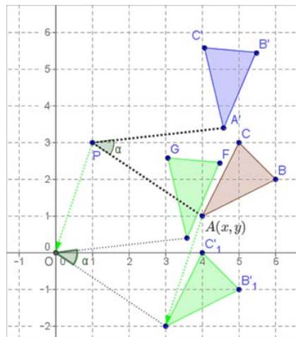
Gambar 47. Rotasi R_{O,\alpha}
