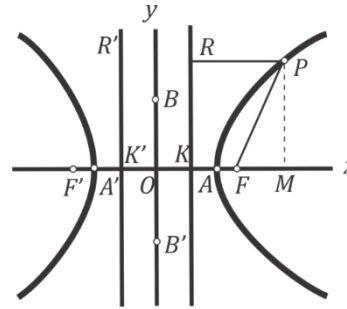
Gambar 109 Definisi Hiperbola
