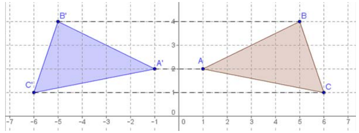
Gambar 51. Refleksi sumbu-y
