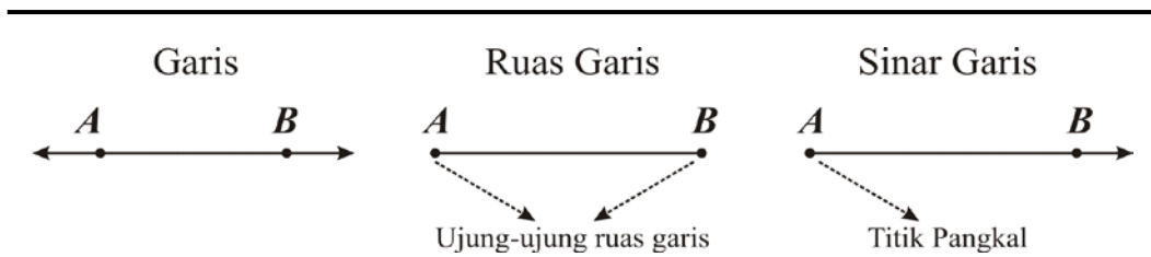
Gambar 2. Garis, Ruas Garis, dan Sinar Garis
