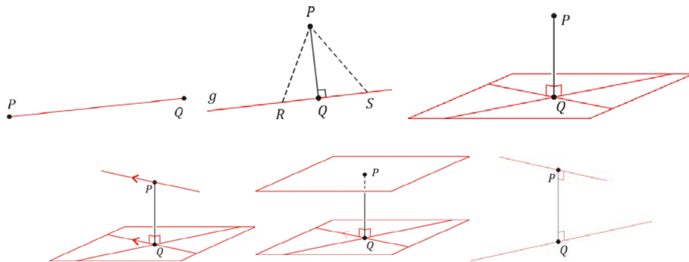
Gambar 88. Jarak antar Objek dalam Geometri
