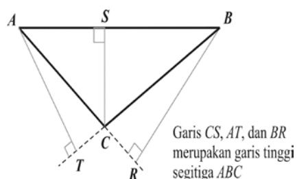
Gambar 18. Garis Tinggi Segitiga
