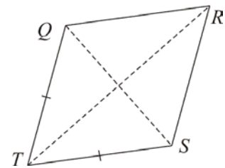
Gambar 28. Belah ketupat
