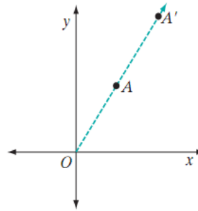
Gambar 57. Dilatasi Berpusat di O
