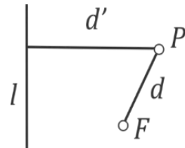
Gambar 99. Definisi irisan kerucut dengan eksentrisitas e = d:d'
