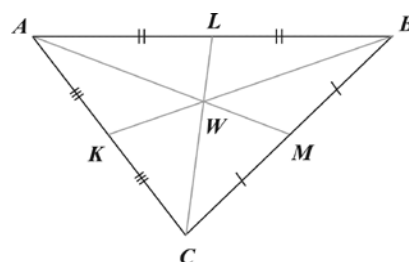
Gambar 19. Garis Berat Segitiga
