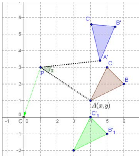
Gambar 46. Translasi ke O
