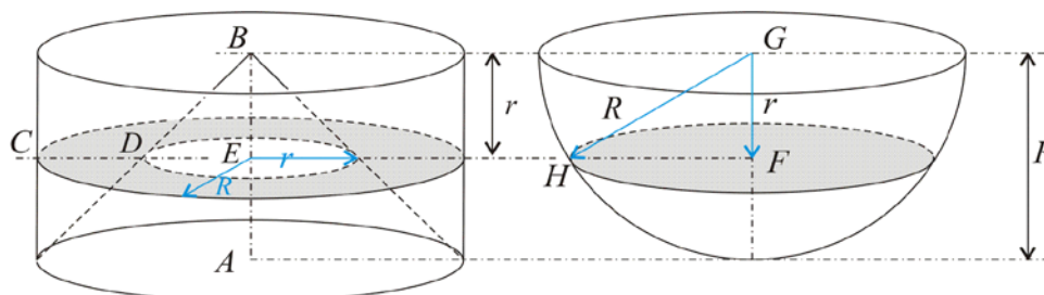
Gambar 82. Volume Bola
