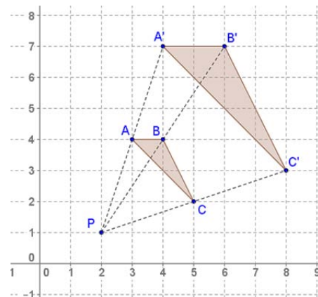
Gambar 56. Dilatasi
