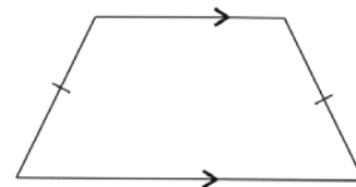
Gambar 31. Trapezium sama kaki
