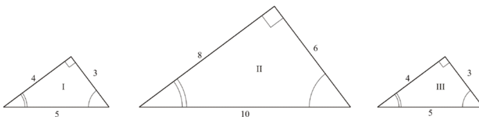
Gambar 21. Kesebangunan
