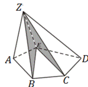
Gambar 74. Volume Limas Segi
