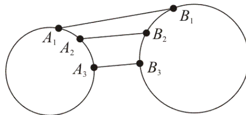
Gambar 87. Jarak dalam Geometri
