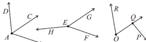
Gambar 5. Hubungan antar Sudut
