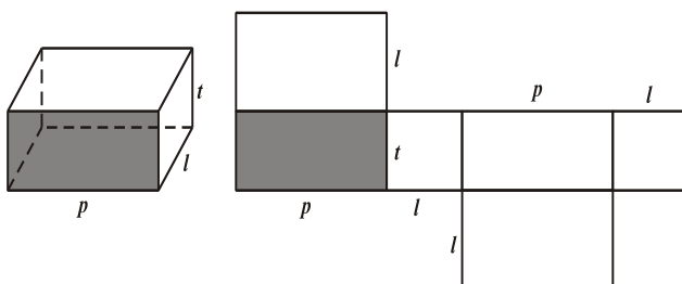
Gambar 61. Luas Permukaan Balok
