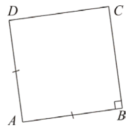
Gambar 29. Persegi
