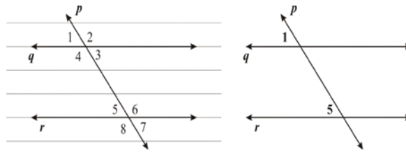
Gambar 9. Postulat 1 garis sejajar
