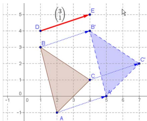
Gambar 43 Translasi
