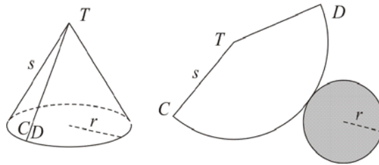
Gambar 80. Luas Permukaan Kerucut
