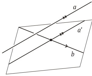
Gambar 90. Sudut antara Dua Garis Bersilangan
