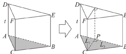
Gambar 67. Volume Prisma Segitiga
