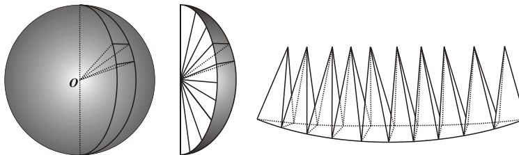
Gambar 83. Luas Permukaan Bola
