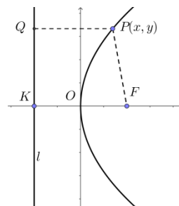
Gambar 101. Parabola dengan puncak di O
