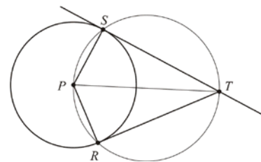
Gambar 39. Ruas Garis Singgung
