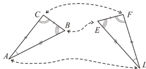
Gambar 12. Dua Segitiga Kongruen
