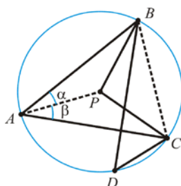
Gambar 37. Hubungan Sudut Pusat dan Sudut Keliling
