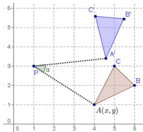
Gambar 45. Rotasi Berpusat di P
