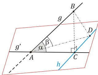
Gambar 91. Sudut antara Garis dan Bidang
