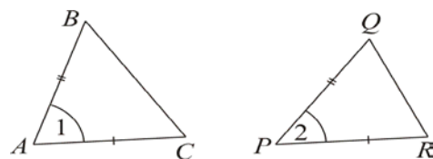
Gambar 15. Ketaksamaan sisi-sisi-
