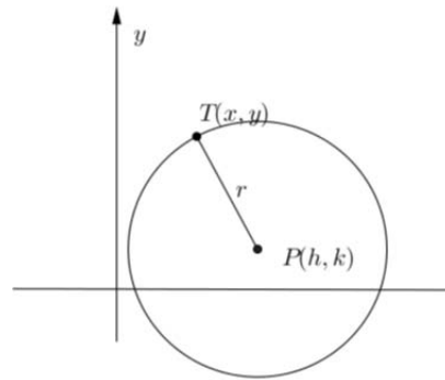
Gambar 113 Lingkaran berpusat di P(h, k)
