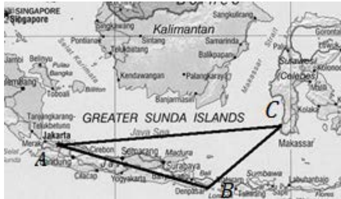
Gambar 13 Sifat Segitiga
