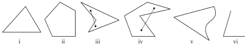
Gambar 26. Poligon dan Bukan Poligon
