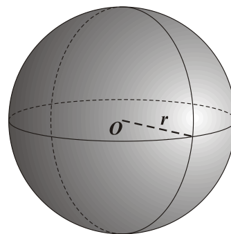
Gambar 81. Bola
