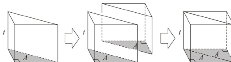
Gambar 66. Volum Prisma Segitiga Siku-siku
