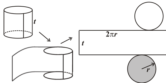
Gambar 77. Bukaan Tabung
