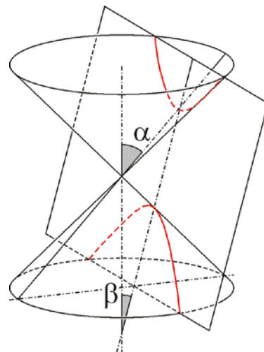
Gambar 98. Irisan kerucut dan bidang berupa hiperbola
