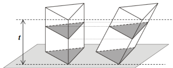
Gambar 70. Volum Prisma Miring
