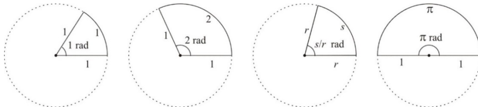
Gambar 4. Satuan sudut dalam Radian
