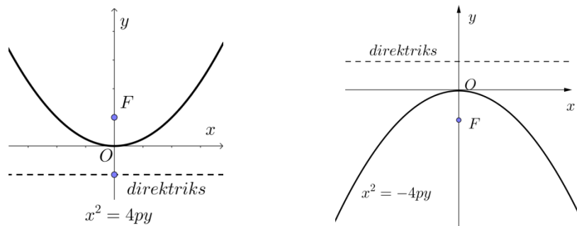
Gambar 103. Parabola dengan sumbu simetri sumbu- y
