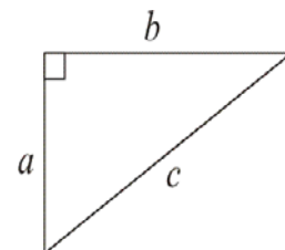
Gambar 23. Teorema Pythagoras
