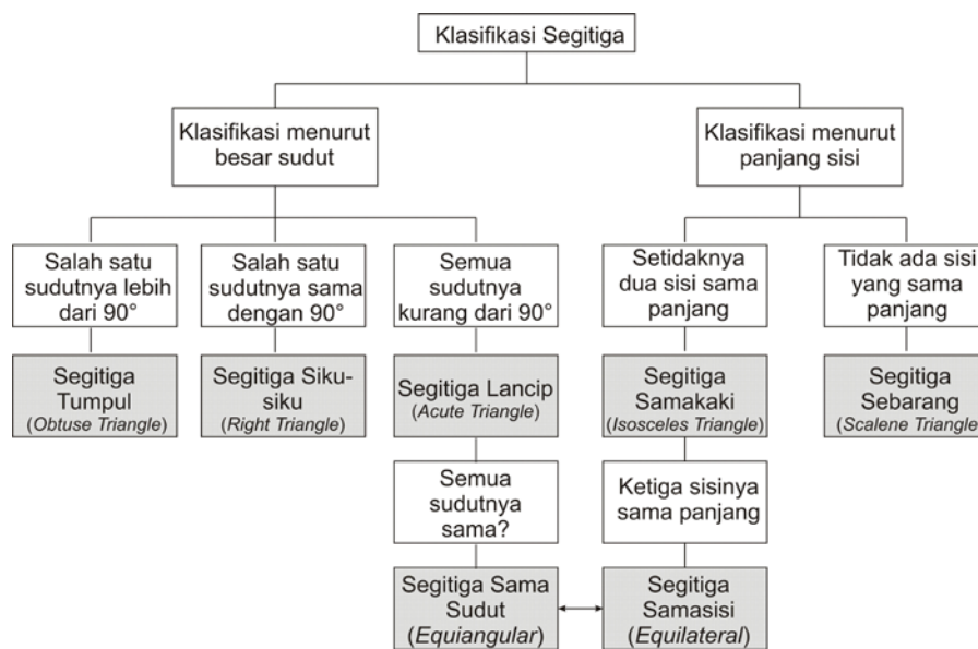
Gambar 11 Bagan Jenis-jenis Segitiga
