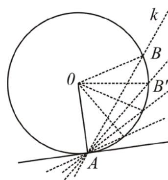
Gambar 38. Garis Singgung
