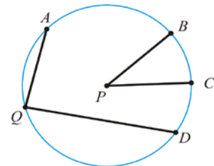
Gambar 36. Sudut Pusat dan Sudut Keliling
