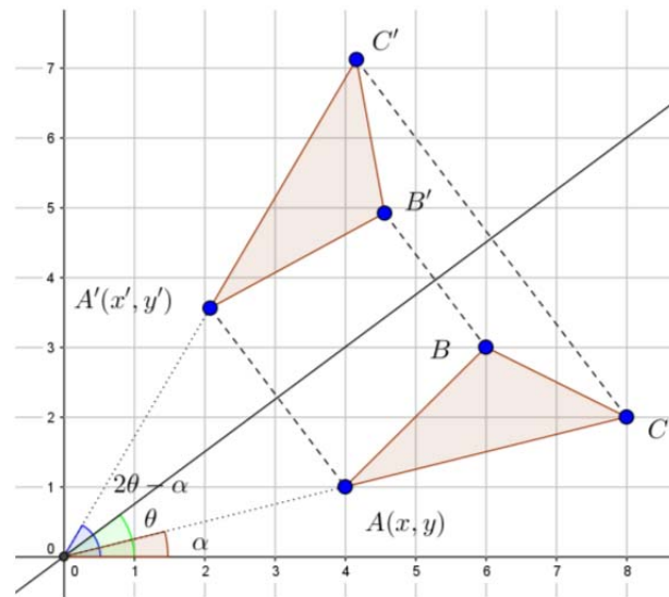
Gambar 53. Refleksi terhadap y = mx
