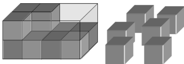
Gambar 63. Volum Balok
