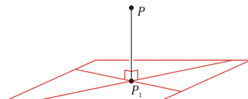
Gambar 84. Proyeksi Titik ke Bidang
