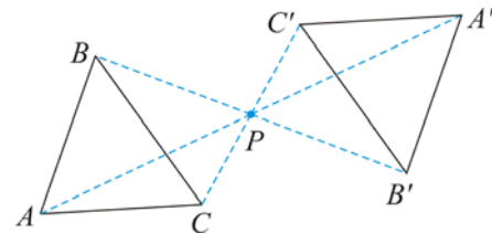
Gambar 54. Refleksi Terhadap Titik
