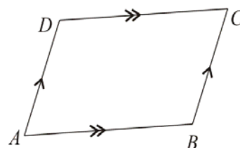
Gambar 27. Jajargenjang
