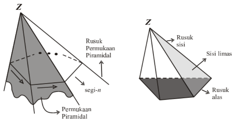
Gambar 72. Limas
