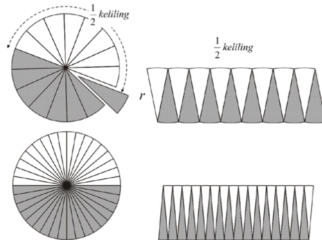
Gambar 35. Luas Lingkaran
