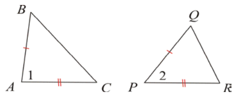
Gambar 14. Ketaksamaan sisi-sudut-sisi
