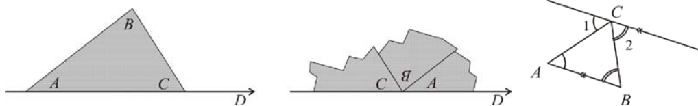
Gambar 16. Menunjukkan Jumlah Sudut Segitiga dan Ilustrasi Bukti
