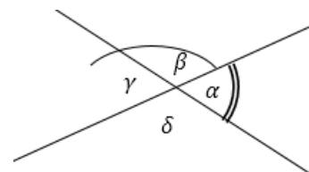
Gambar 89. Sudut antara Dua Garis Berpotongan
