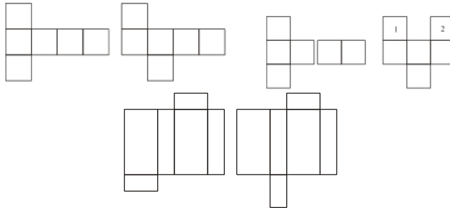
Gambar 62 Jaring-jaring dan bukan jaring-jaring
