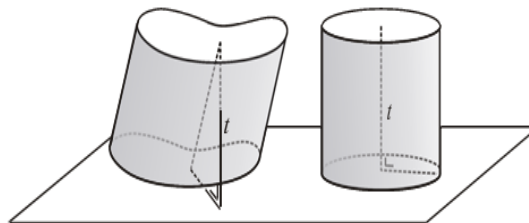
Gambar 76. Tabung
