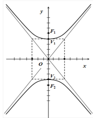
Gambar 111 Hiperbola dengan sumbu nyata sumbu- y
