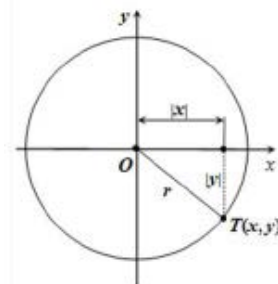
Gambar 112. Lingkaran berpusat di O(0,0) dan berjari-jari r
