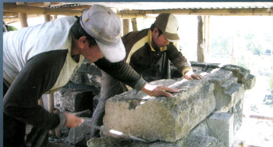
Reposisi Komponen Batu Kulit
