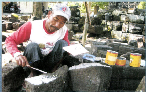
Penyambungan Batu Menggunakan Epoxy Rigit Bonding (Sikadur) dan Water Repellent
