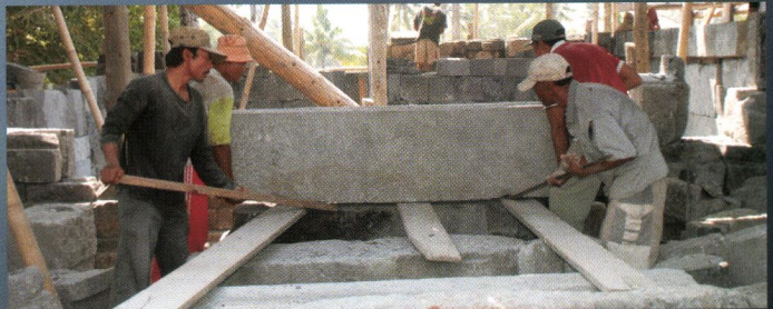
Pemasangan Batu Dorpel Candi
