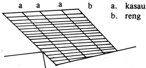
Gambar 11 Pemasangan kasau dan reng
