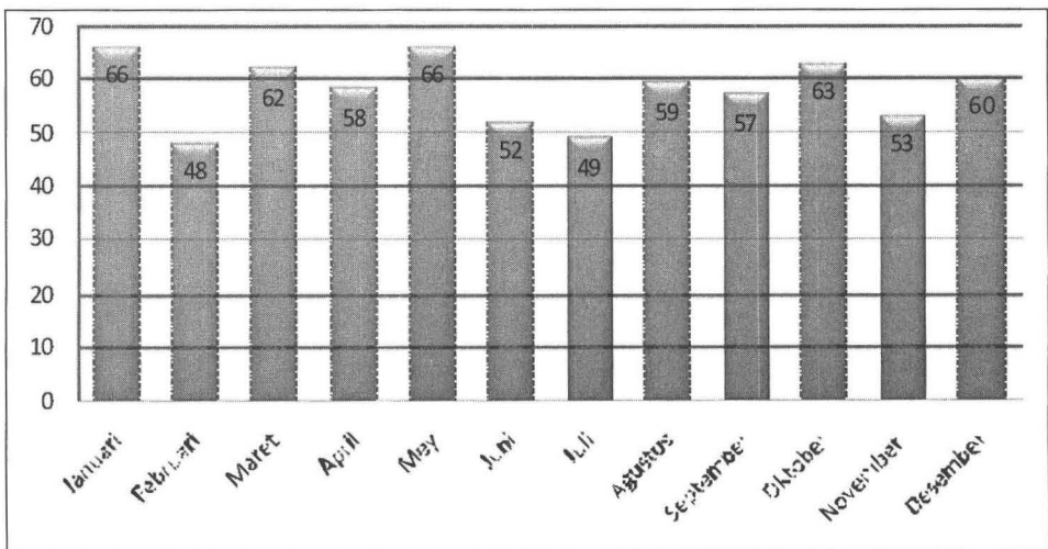
Grafik 1. Rata-rata Penyinaran Matahari Tahun 2012
