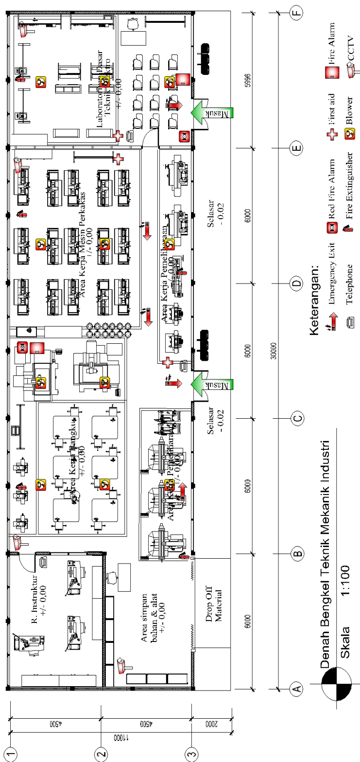
Gambar 21. Visualisasi 2D ruang praktik siswa kompetensi keahlian teknik mekanik industri
