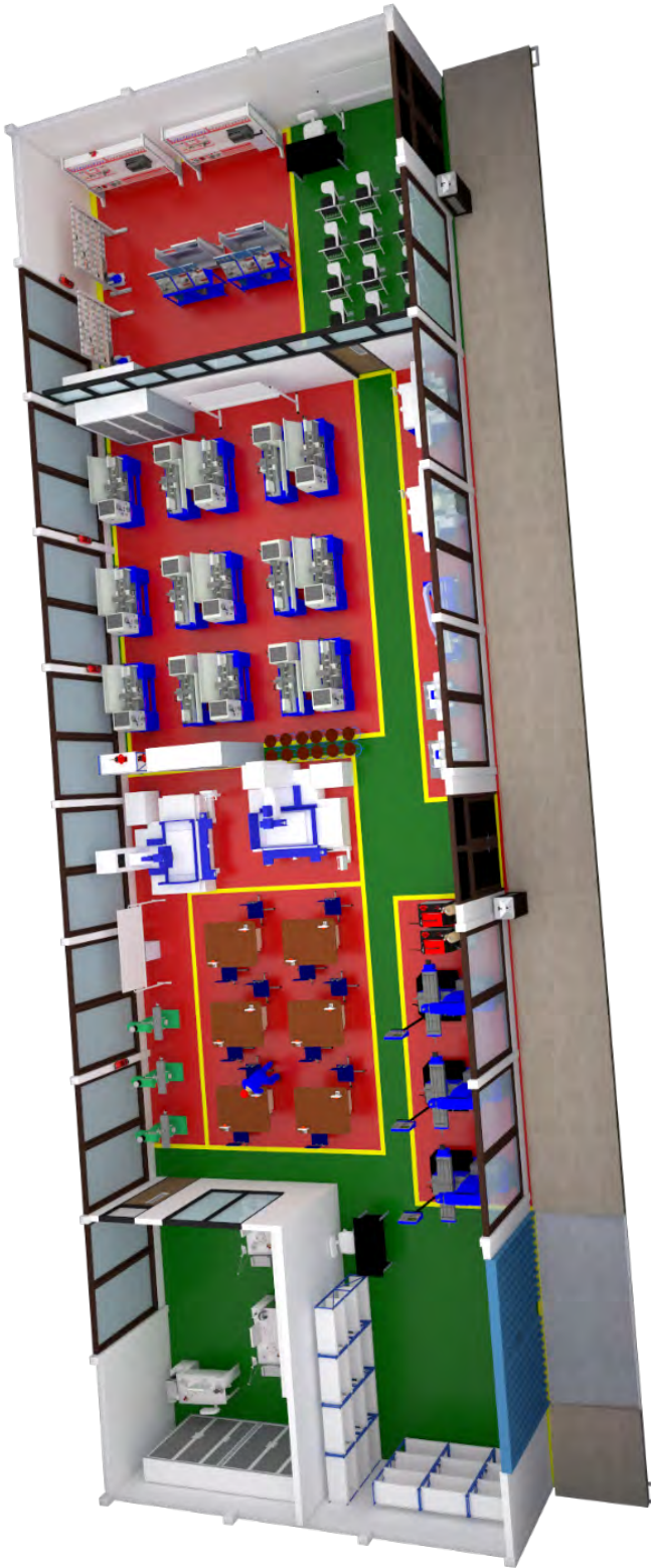
Gambar 22. Visualisasi 3D ruang praktik siswa kompetensi keahlian teknik mekanik industri tampak 1
