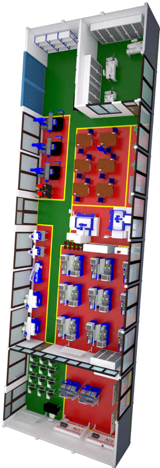
Gambar 23. Visualisasi 3D ruang praktik siswa kompetensi keahlian teknik mekanik industri tampak 2
