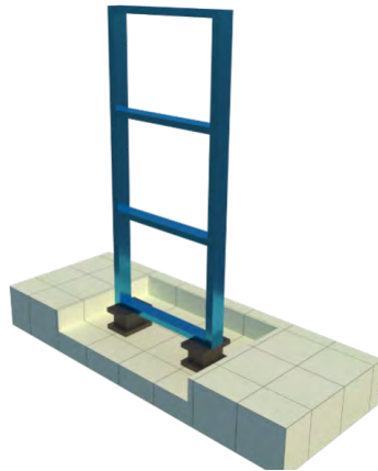
Gambar 8. Ilustrasi struktur yang diberikan isolation bearing
