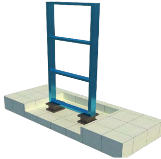
Gambar 8. Ilustrasi struktur yang diberikan isolation bearing
