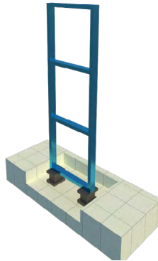
Gambar 8. Ilustrasi struktur yang diberikan isolation bearing
