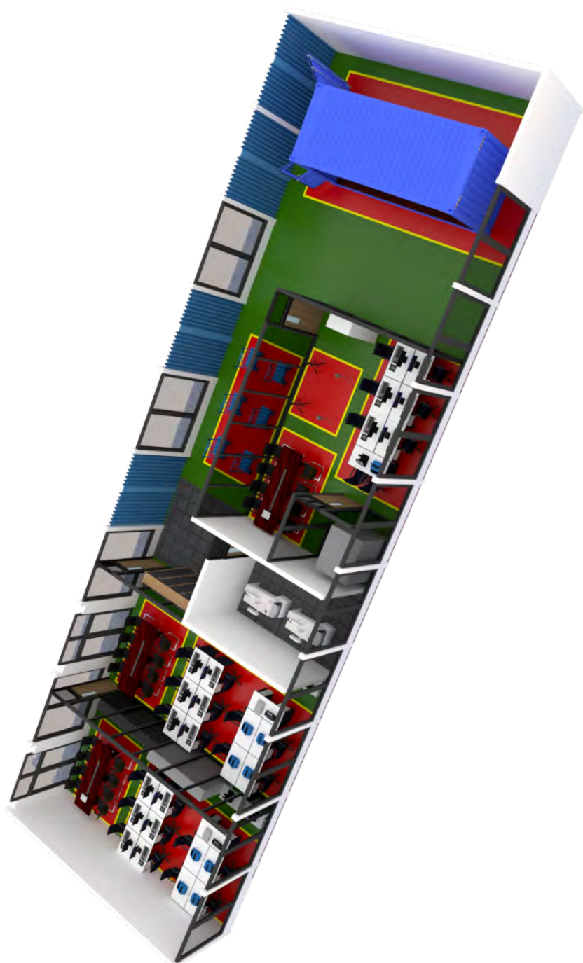
Gambar 23. Visualisasi 3D ruang praktik siswa kompetensi keahlian manajemen logistik tampak 2
