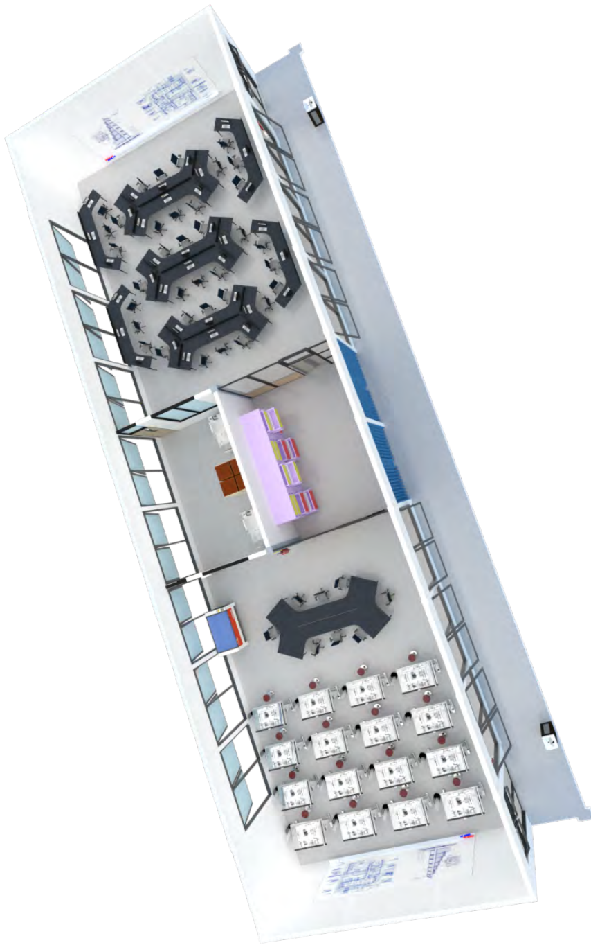
Gambar 22. Visualisasi 3D ruang praktik siswa kompetensi keahlian desain pemodelan dan informasi bangunan tampak 1
