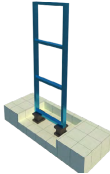
Gambar 8. Ilustrasi struktur yang diberikan isolation bearing
