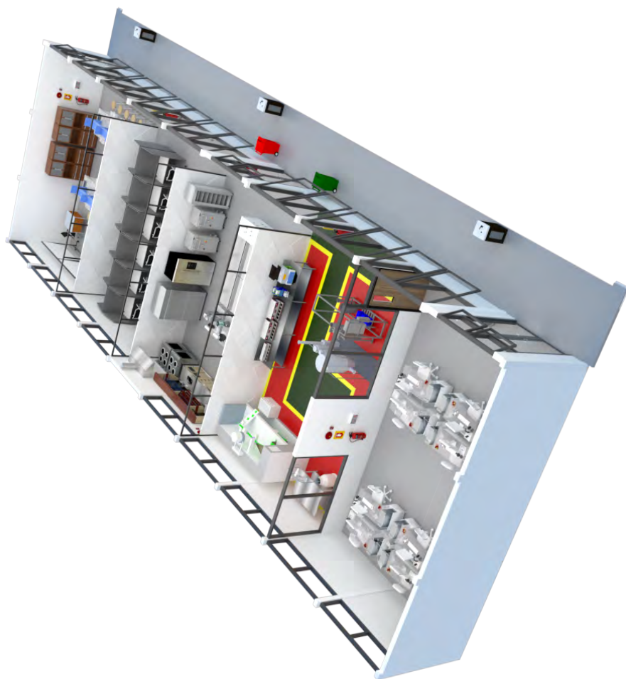
Gambar 22. Visualisasi 3D ruang praktik siswa kompetensi keahlian agribisnis pengolahan hasil pertanian tampak 1.
