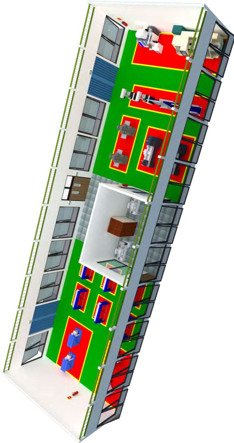
Gambar 23. Visualisasi 3D ruang praktik siswa kompetensi keahlian teknik pemesinan kapal tampak 2
