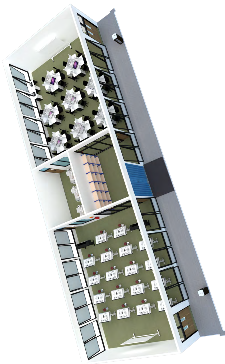
Gambar 22. Visualisasi 3D ruang praktik siswa kompetensi keahlian desain dan rancang bangun kapal tampak 1
