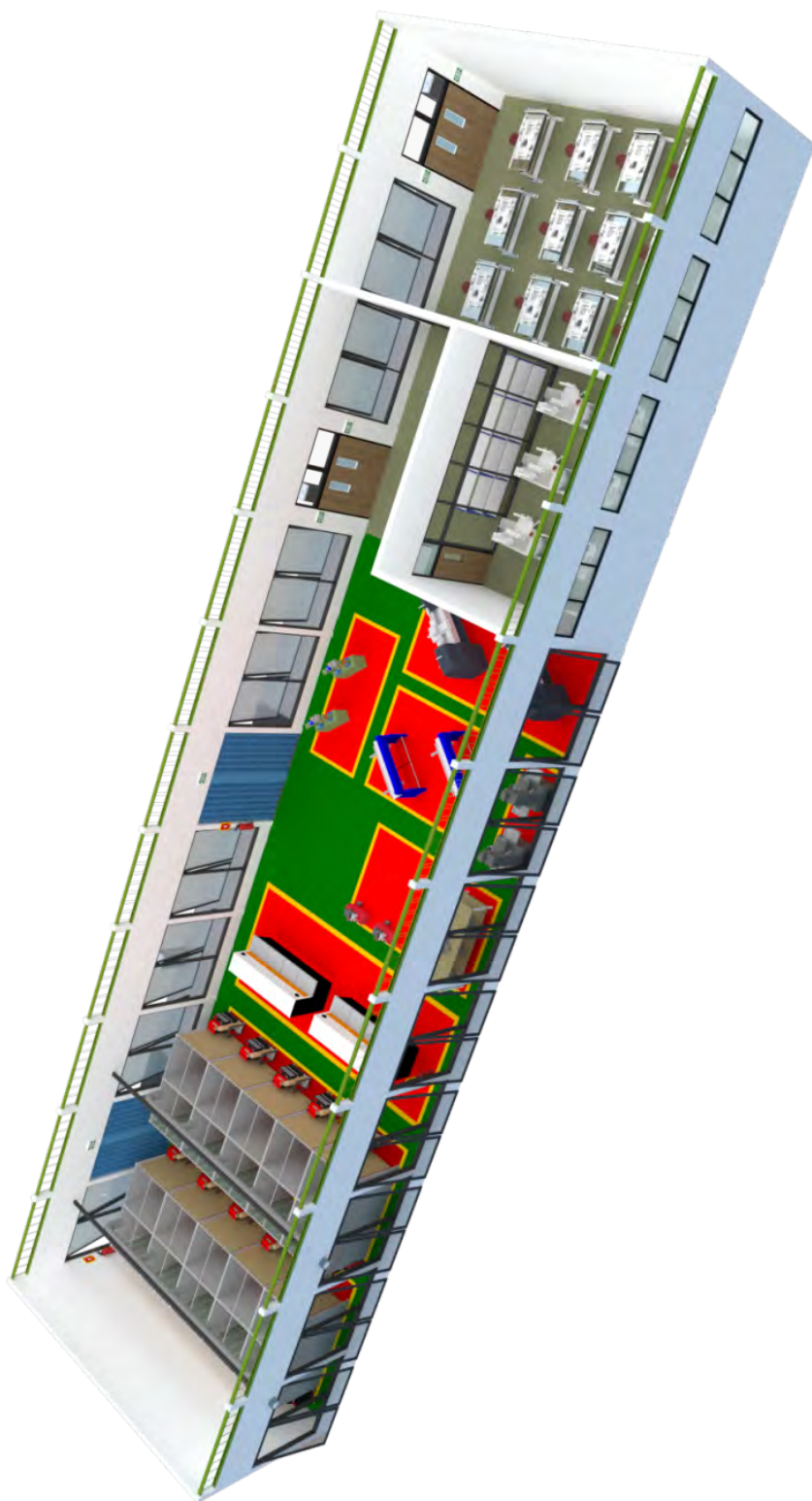
Gambar 23. Visualisasi 3D ruang praktik siswa kompetensi keahlian konstruksi kapal baja tampak 2
