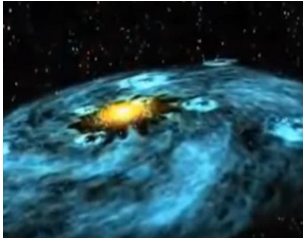
Gambar 3. Teori Nebula
