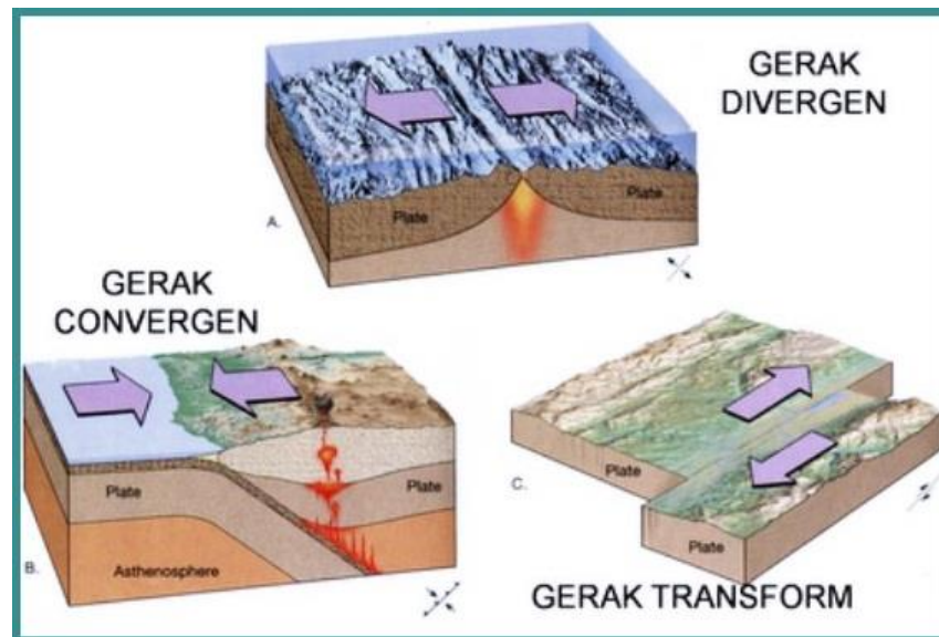
Gambar 7. Gerak Lempeng Tektonik
