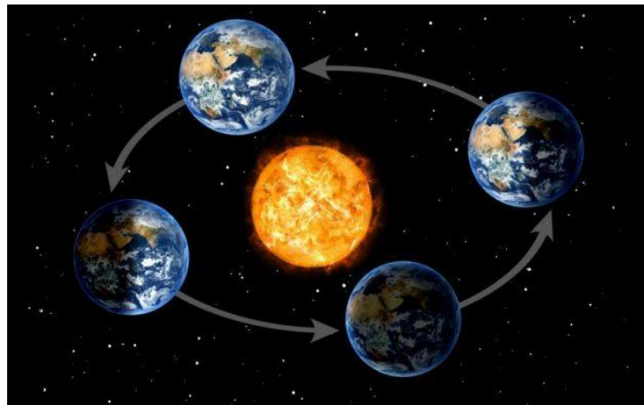
Gambar 9. Revolusi Bumi
