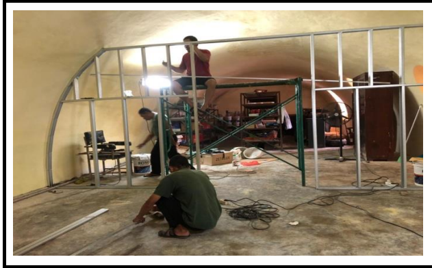
FOTO KEGIATAN PEMASANGAN RANGKA PARTISI BAGIAN BAWAH 100%
