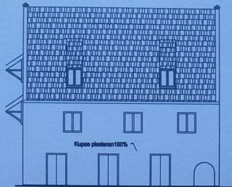
TAMPAK SELATAN
