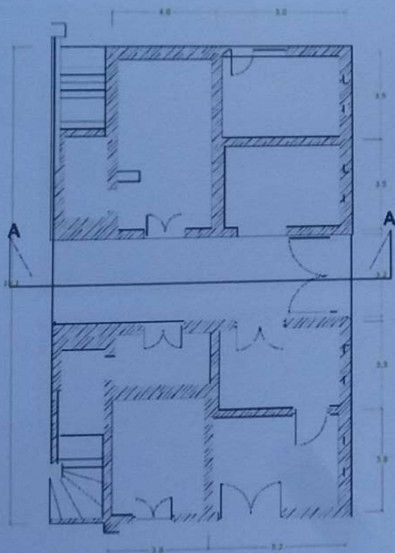
Lantai I BANGUNAN A KOMP. BALANG NIPA Skala 1 : 100
