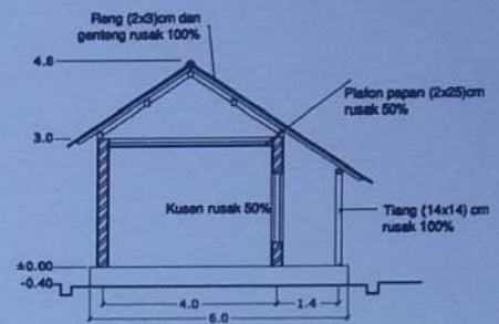
POTONGAN B-B GEDUNG J SKALA 1 : 100
