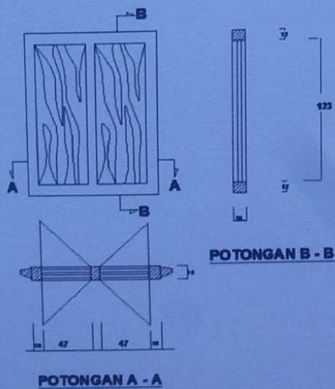
DETAIL DAUN JENDELA LT.III Skala 1 : 30
