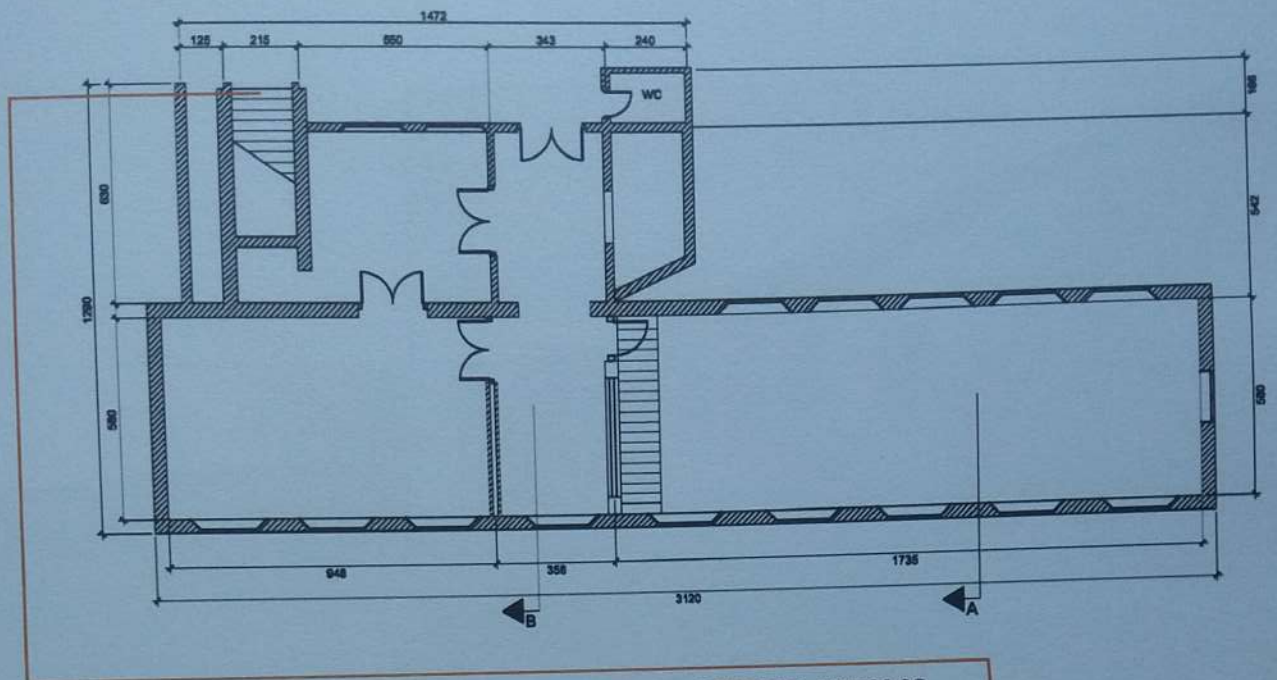
DENAH LANTAI 02 Skala 1 : 120
