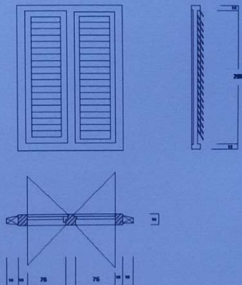
DETAIL DAUN JENDELA LT.II Skala 1 : 30
