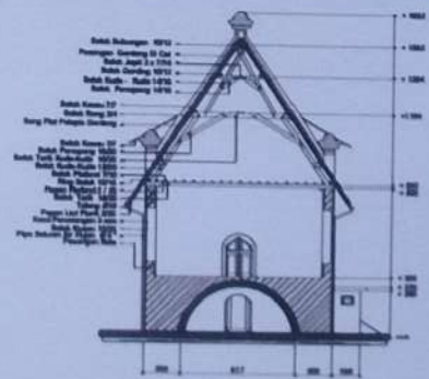
POTONGAN A
