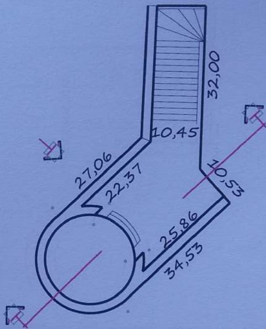
BALAI PELESTARIAN CAGAR BUDAYA UDENAH EXISTING BASTION 4 LT. ATAS
