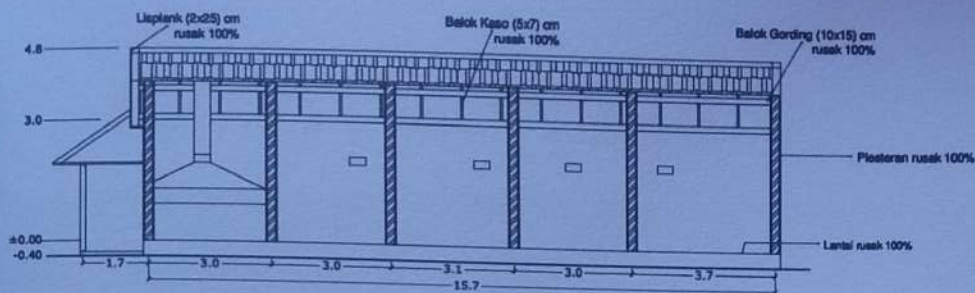
POTONGAN A-A GEDUNG J SKALA 1 : 100
