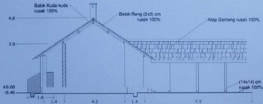
POTONGAN B-B GEDUNG B SKALA 1 : 100
