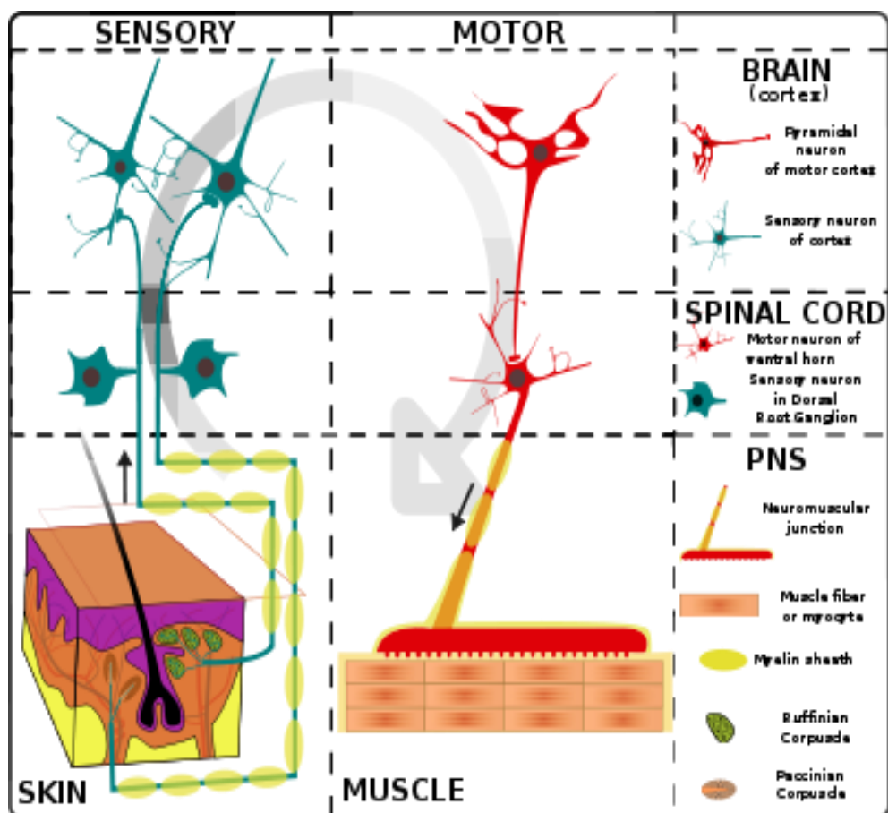
Gambar 38. neuron pada spinsl cord. (Sumber: Cambell et al. 1999)
