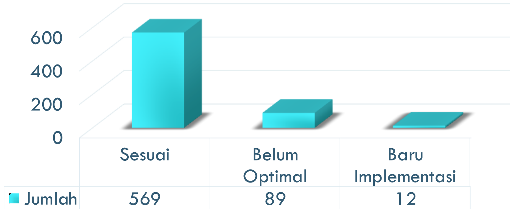
Evaluasi BW
