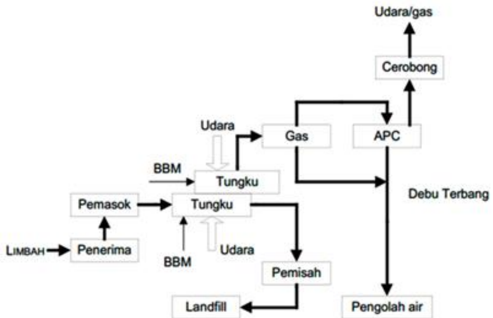
Gambar 10. Prinsip Proses Insinerasi
