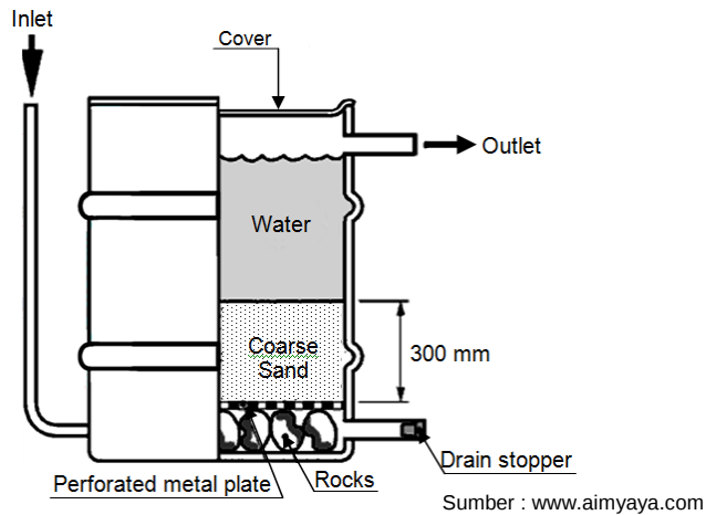
Gambar 7. Skema Penyaringan Pasir Cepat
