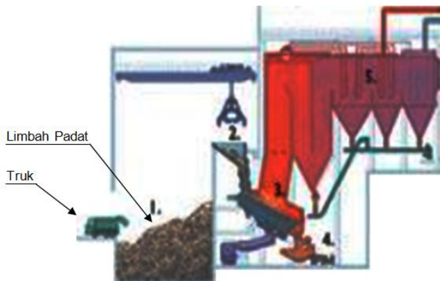
Gambar 5. Cara Kerja Pengumpulan dan Pembakaran Limbah Padat
