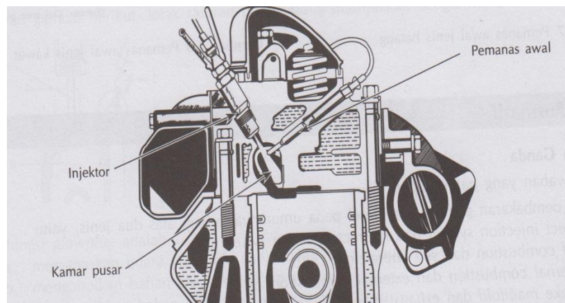
Gambar 33. Busi pijar/ glowplug yang dipasang pada sistem kamar puser.
