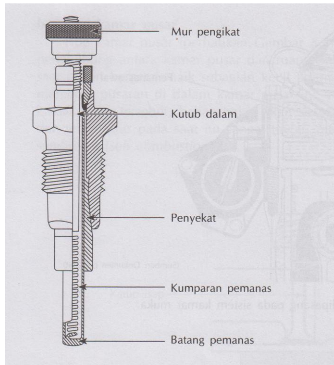
Gambar 37. Pemanas awal jenis kawat.
