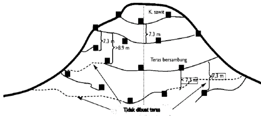
Gambar 34. Pemancangan teras kontur dengan sistem Violle
