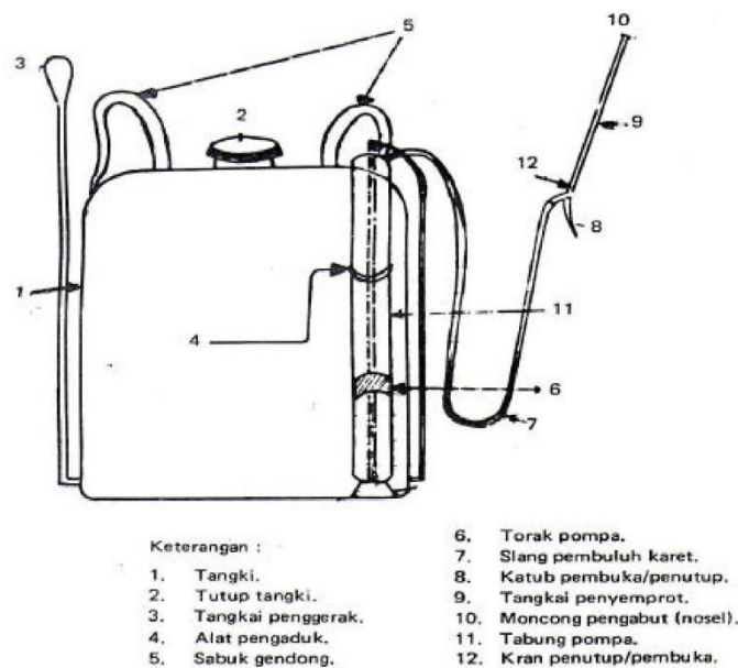
Gambar 37. Knapsack Sprayer dan bagian-bagiannya (Hardjosentono,1996)
