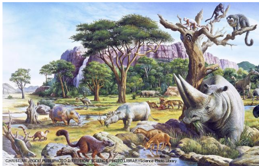
Gambar 2.20 Kehidupan pada kala paleosen. Sumber :
