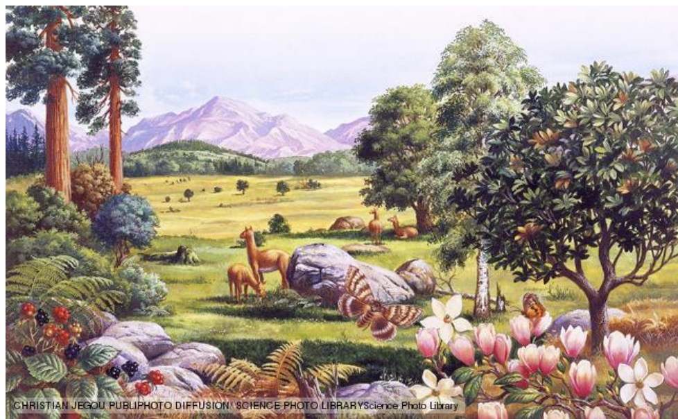
Gambar 2.24 Kehidupan pada kala pliosen. Sumber :
