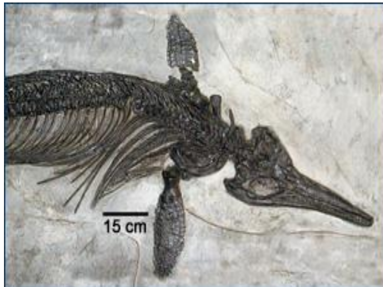
Gambar 2.14 Fosil Ichthyosaurus intermedius pada jaman Jura. Sumber : http://www.ucmp.berkeley.edu/mesozoic/jurassic/jurassic.php
