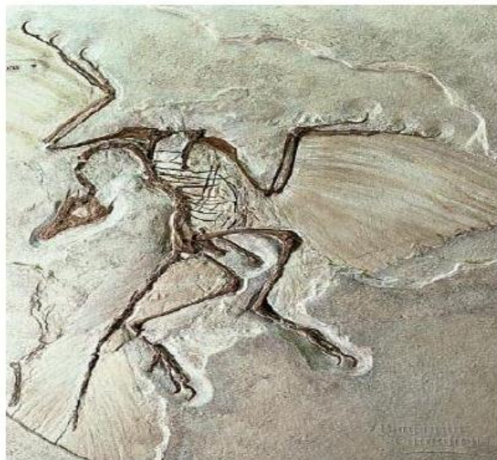
Gambar 1.7. Fosil Archaeopteryx lithographica , berumur Jura, memiliki rangka reptil yang didalamnya memiliki jari-jari dengan cakar pada sayapnya, susunan tulang belakang yang menerus hingga ke bagian ekor, serta memiliki gigi, akan tetapi tubuh binatang ini ditutupi oleh bulu.
