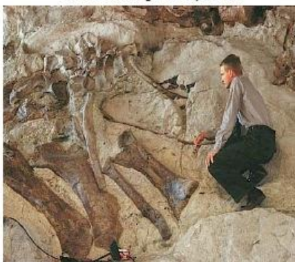
Fosil dari hasil organismenya sendiri
