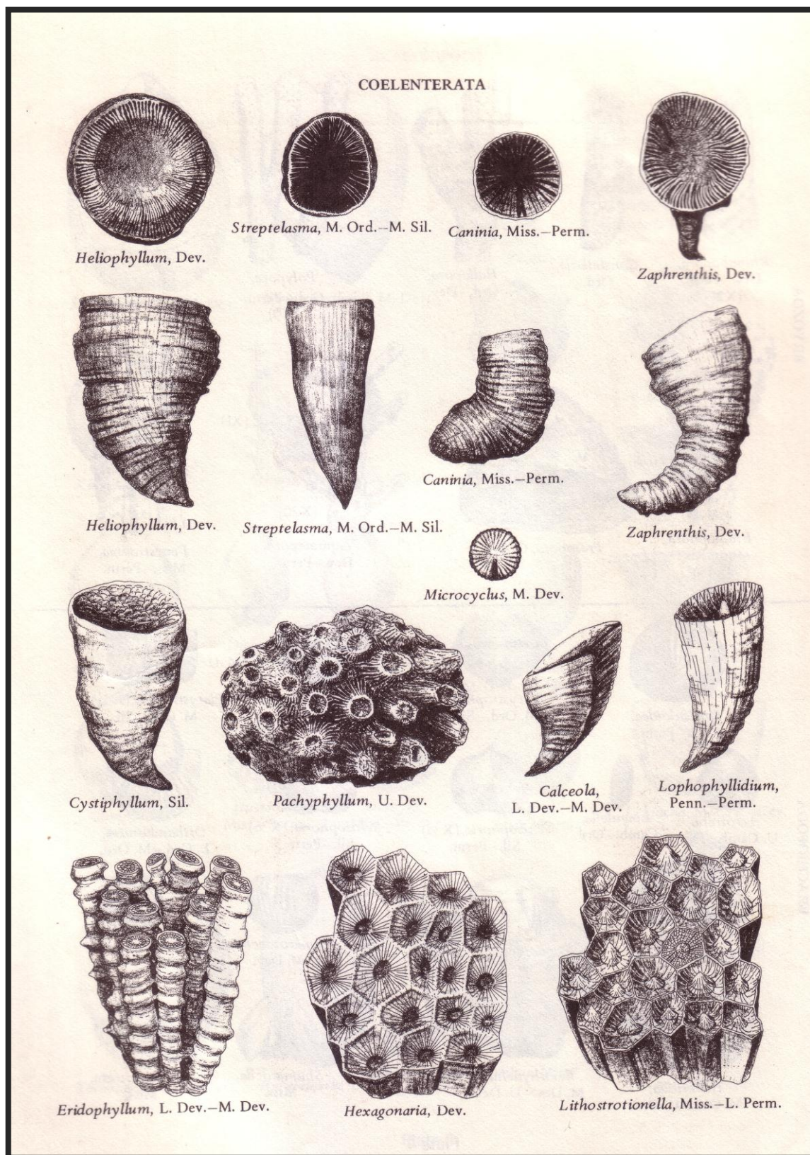
Gambar 3.16. Berbagai contoh fosil coelenterata . Sumber : Interpreting earth history
