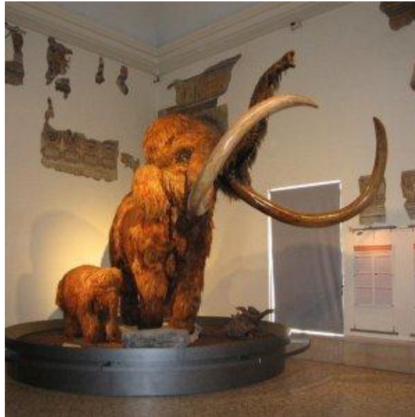
Gambar 1.10. Fosil Mammoth. Sumber : www.newsystype.com
