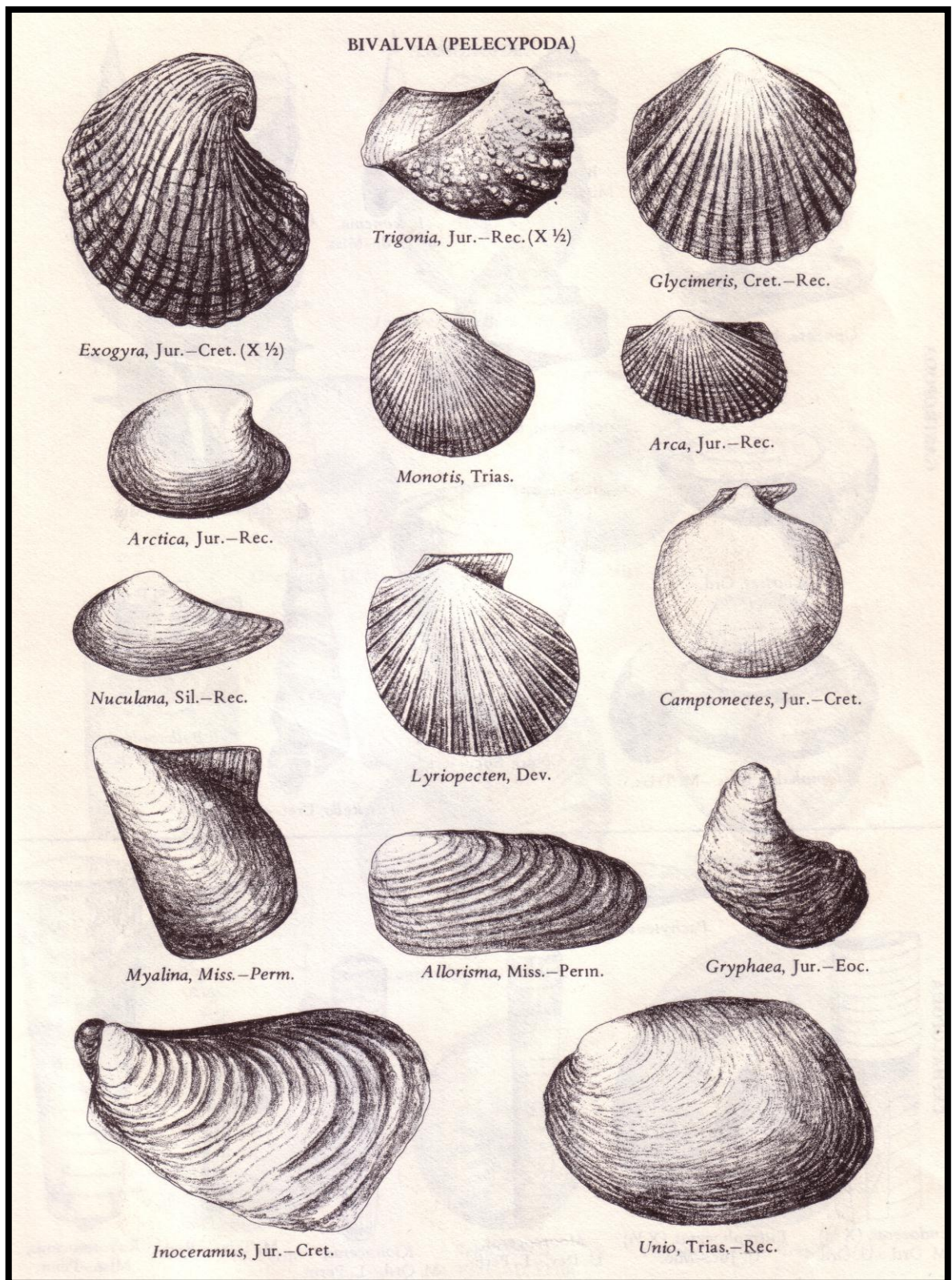
Gambar 3.7. Contoh Fossil Pelecypoda. Sumber : Interpreting earth history Morris s. petersen
