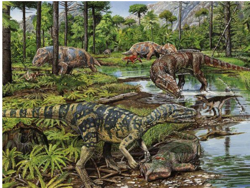
Gambar 2.13 Kehidupan pada jaman Trias. Sumber : science.nationalgeographic.com
