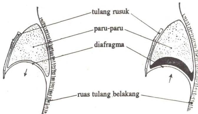
GAMBAR No. 1 Posisi diafragma sebelum pengambilan napas Bagian yang hitam menunjukkan penambahan volume paru-paru
